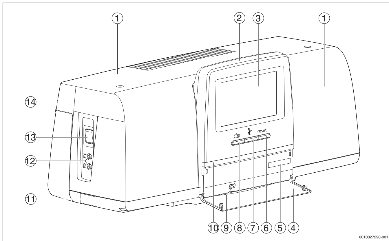
Bild 1 Übersicht Regelgerät
