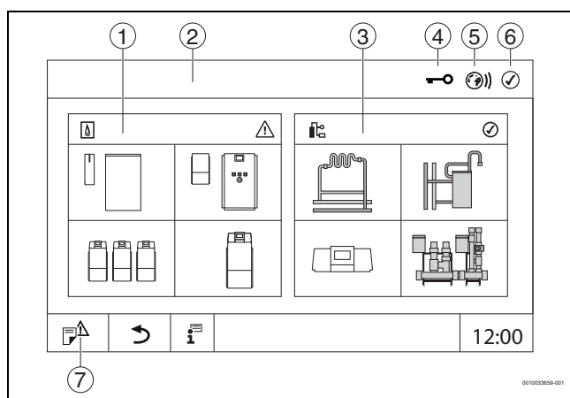
Bild 2 Systemübersicht (Beispiel)
