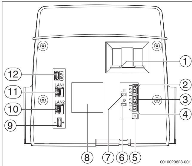
Bild 7 Anschlüsse Bedieneinheit
