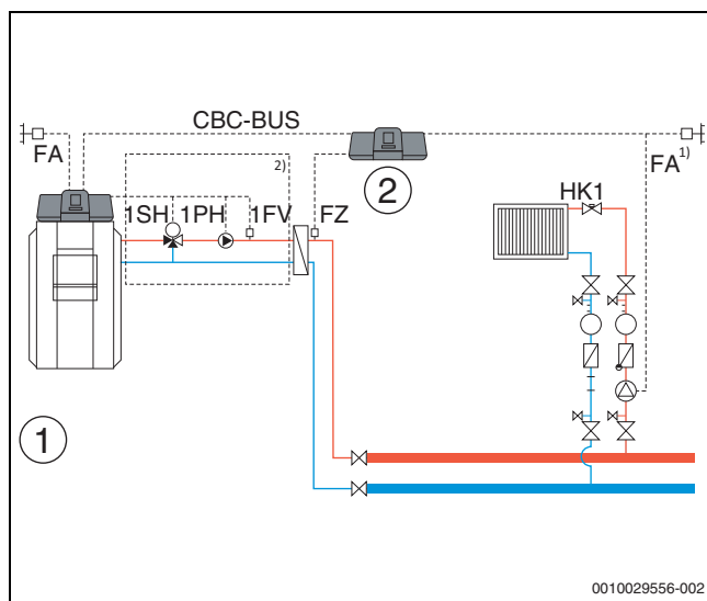
Bild 30 Variante 3: Unterstation mit Vormischfunktion, Kompensation Wärmeverluste über FZ, Lastbegrenzung und Heizbetrieb bei Kommunikationsverlust
