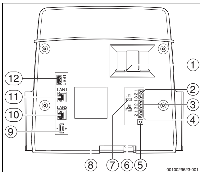
Bild 20 Rückseite Bedieneinheit
