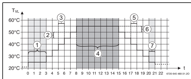
Bild 39 Estrichtrocknung
