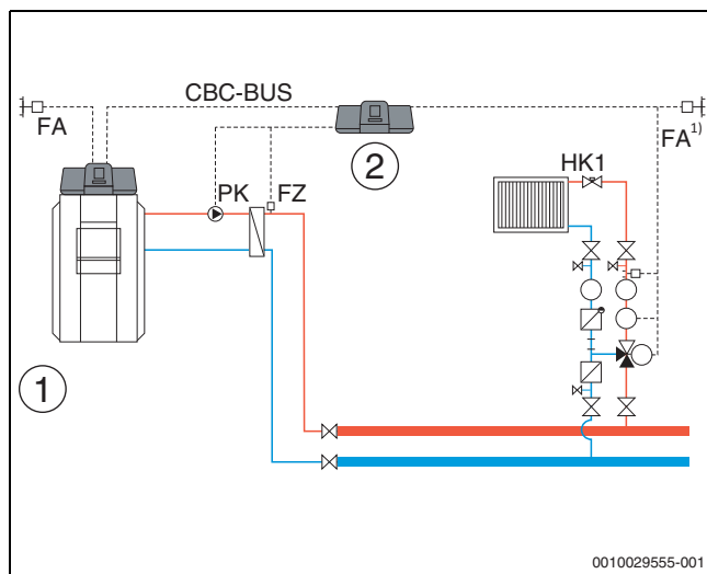
Bild 29 Variante 2: Unterstation mit Kompensation Wärmeverluste über FZ, Lastbegrenzung
