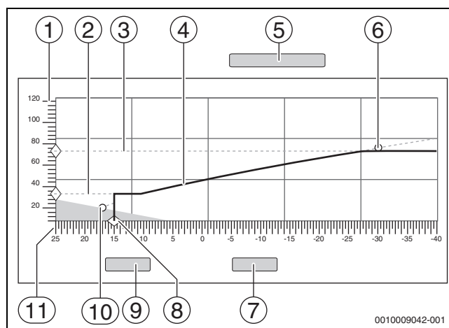
Bild 38 Heizkurve
