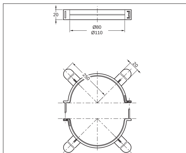
Bild 141 Abstandshalter für Abgasleitung im Schacht (Maße in mm)
