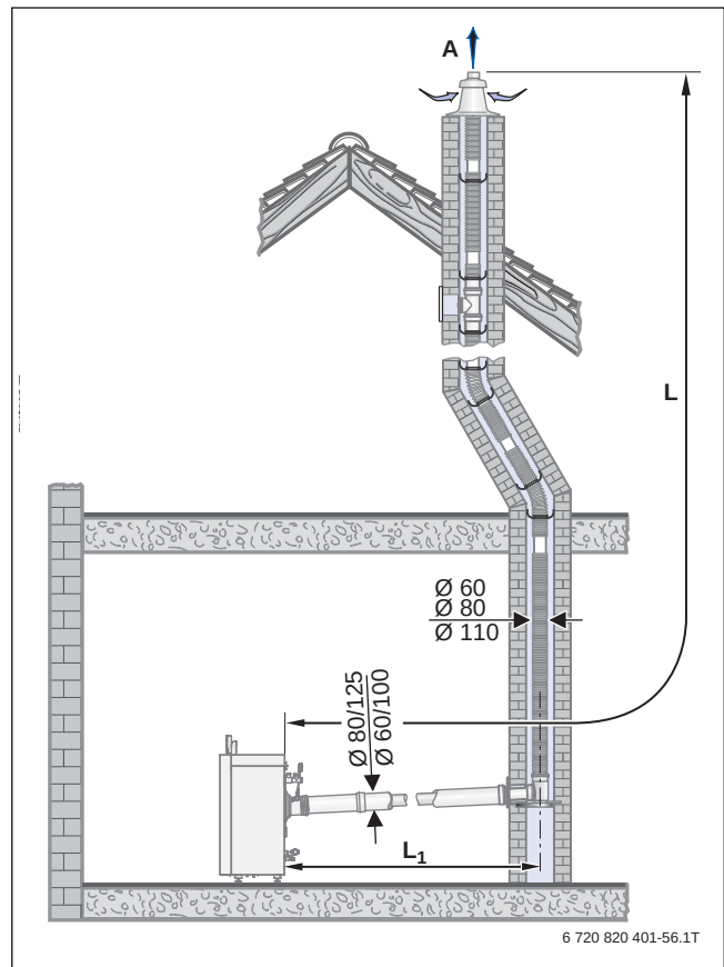
Bild 118 Montagevarianten mit dem Bausatz GA-K + ÜB-Flex
