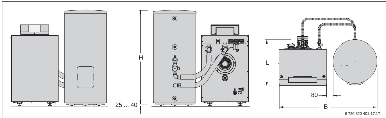
Bild 12 Abmessungen Logano plus KB192i mit Logamatic und Logalux SU (Maße in mm)
