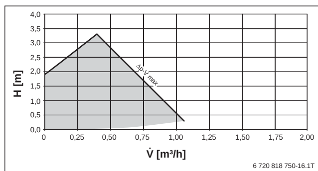
Bild 69 Restförderhöhe HSM15 V3: Dp-V
