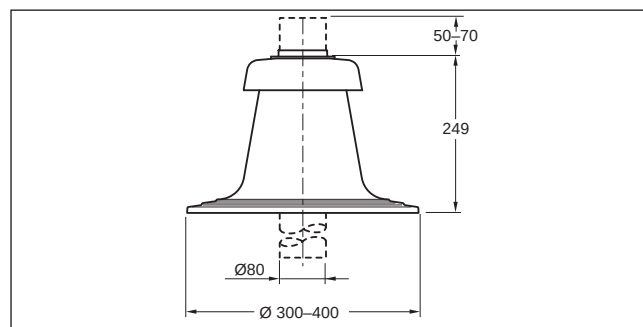
Bild 139 Schachtabdeckung für 80 mm (Maße in mm)
