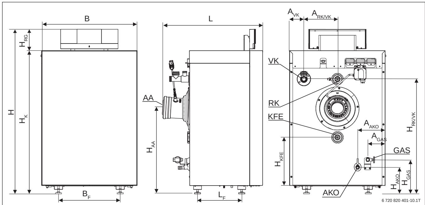
Bild 10 Abmessungen und Anschlüsse für Logano plus KB192i (Maße in mm)
