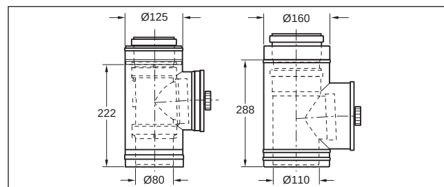
Bild 154 Konzentrisches Rohr mit Prüföffnung aus Edelstahl (Maße in mm)
