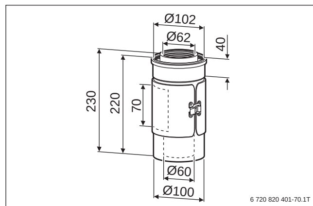
Bild 151 Konzentrisches Rohr mit Prüföffnung Ø 60/100 (Maße in mm)
