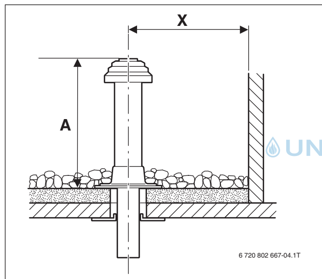
Bild 101 Mindestabstände Flachdach
