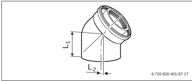
Bild 155 Konzentrischer Bogen Ø 60/100 (Maße → Tabelle 77)
