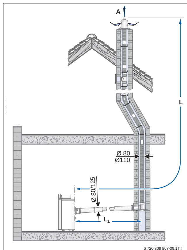
Bild 128 Montagevarianten mit dem Bausatz GA-K + ÜB-Flex
