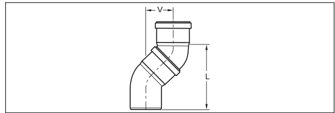
Bild 132 Versatzmaße Bogen
