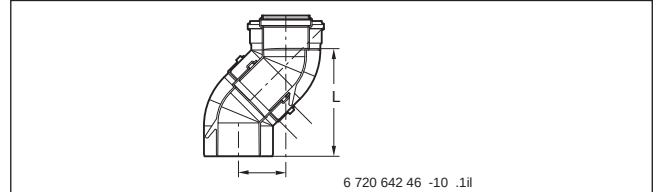
Bild 159 Versatzmaße konzentrischer Bogen Ø 80/125 (Maße → Tabelle 78)
