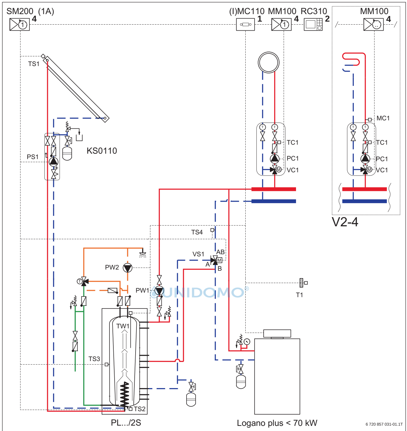
Bild 30 Anlagenbeispiel: Logano plus KB192i/GB212 mit einem gemischten Heizkreis und Kombispeicher Logalux PL.../2S (Abkürzungsverzeichnis → S. 40)
