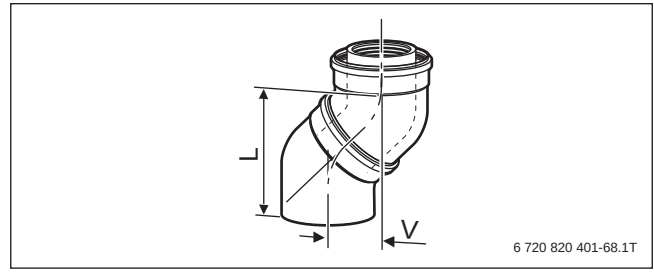
Bild 158 Versatzmaße konzentrischer Bogen Ø 60/100 (Maße → Tabelle 78)
