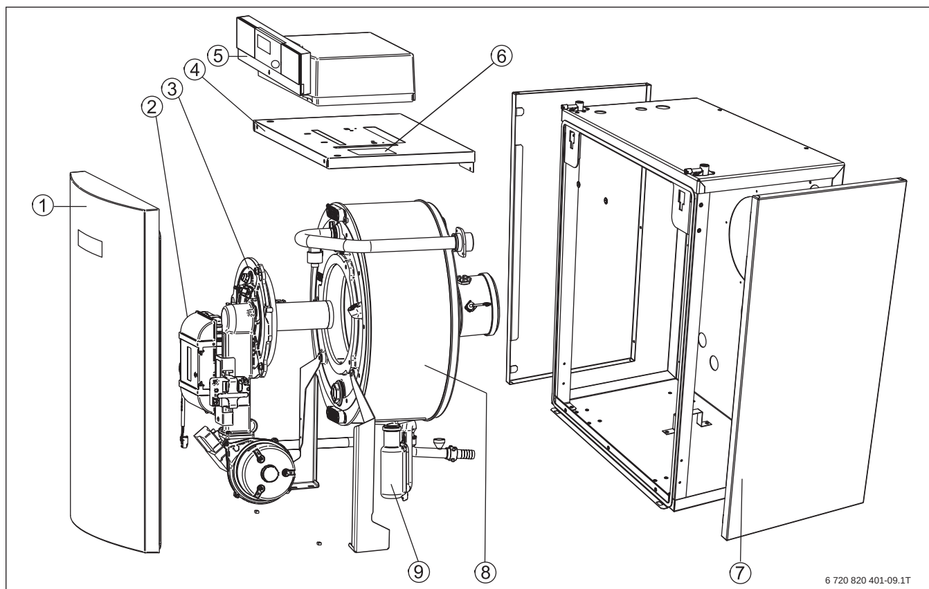
Bild 9 Logano plus GB212
