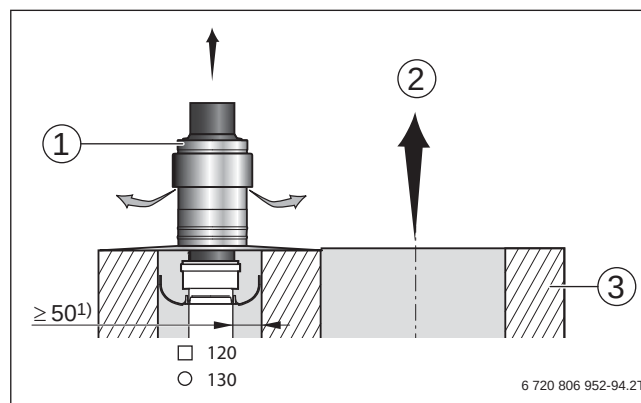
Bild 107 Mindestmaße des Schachtquerschnitts und der Schachtmündung in Verbindung mit Feuerstätten für feste Brennstoffe (Maße in mm)
