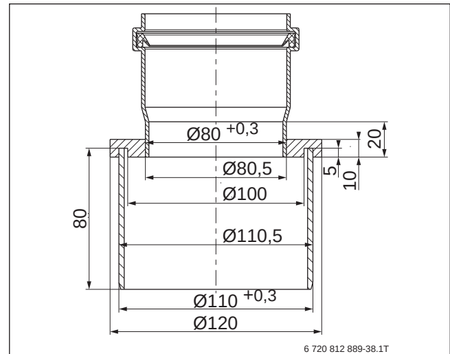
Bild 178 Zentrische Reduktion DN 110 auf DN 80
