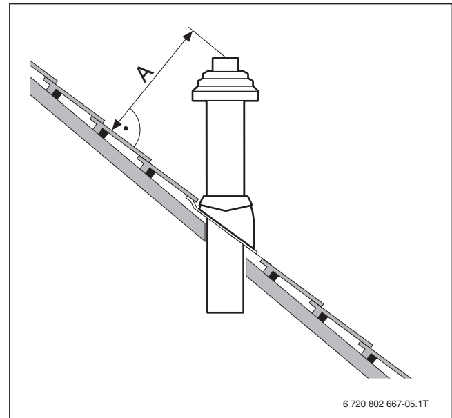
Bild 102 Mindestabstände Schrägdach
