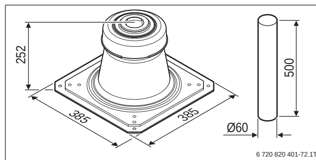
Bild 138 Schachtabdeckung für 60 mm, Kunststoff (Maße in mm)
