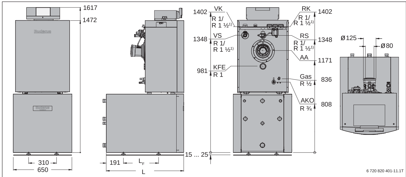
Bild 14 Abmessungen Logano plus GB212 mit Logamatic und Logalux L/2R (Maße in mm)
