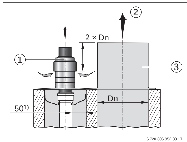
Bild 106 Schachtmündung für die Abgasleitung des Bau-satzes GA-K in Verbindung mit Feuerstätten für feste Brennstoffe (Maße in mm)
