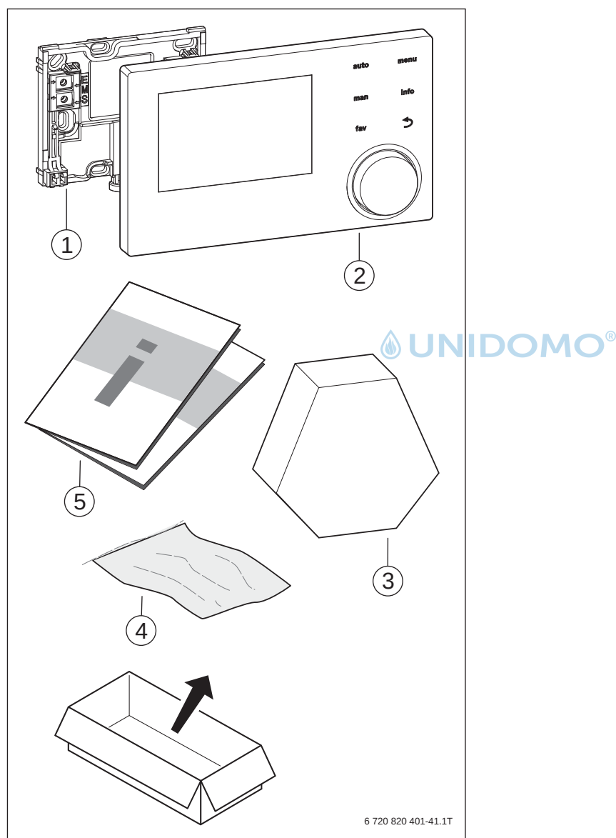
Bild 42 Lieferumfang RC310
