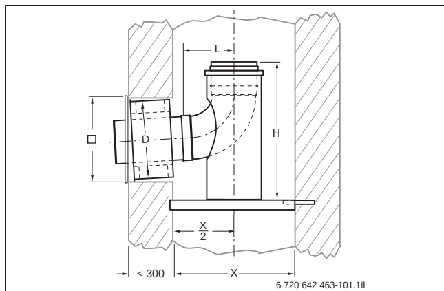
Bild 171 Schornsteinanschluss (Maße in mm)
