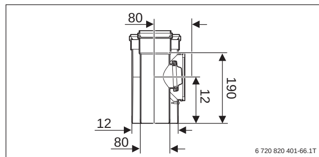
Bild 152 Konzentrisches Rohr mit Prüföffnung Ø 80/125 (Maße in mm)
