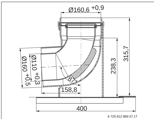
Bild 177 Stützbogen für DO-S in DN 110/160
