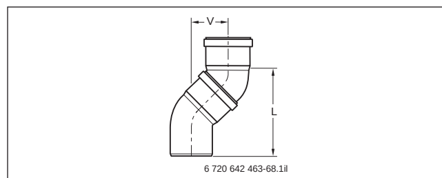
Bild 174 Versatzmaße
