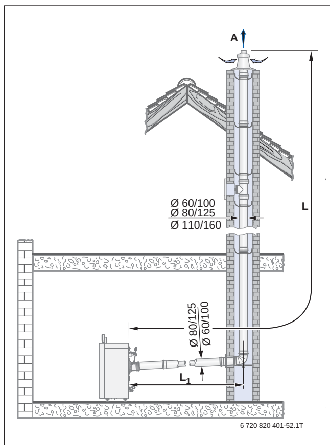
Bild 114 Montagevarianten mit dem Bausatz DO-S
