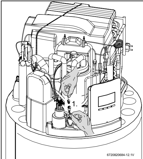
Bild 50 Gebläse-Anschlusskabel
