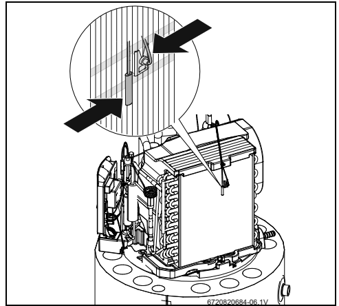
Bild 10 Temperaturfühler (Lamellen des Verdampfers + Ansaugluft)
