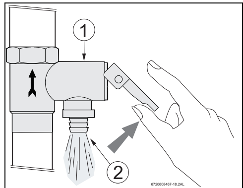
Bild 55 Sicherheitsventil
