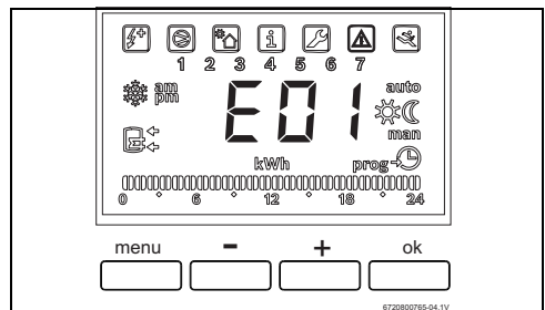
Bild 45 Störungsanzeige mit zugehörigem Fehlercode
