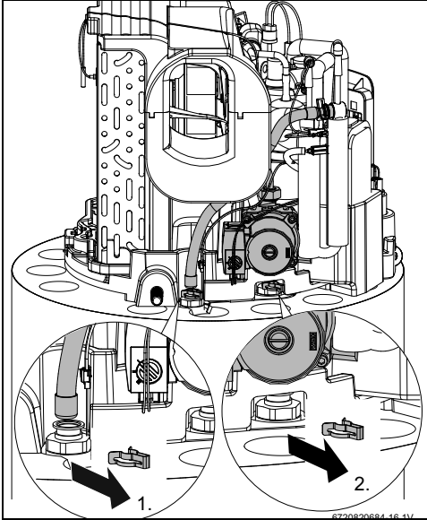
Bild 53 Haltefeder abnehmen
