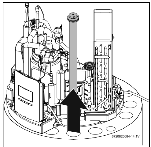
Bild 52 Kontrolle des Zustands der Magnesium-Anode
