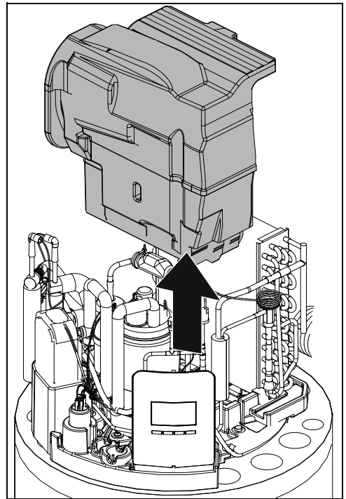
Bild 51 Baugruppe Luftführung und Gebläse entfernen.
