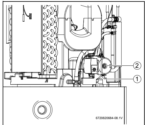
Bild 13 Umwälzpumpe
