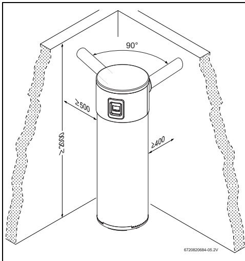
Bild 9 Empfohlene Mindestabstände (mm)
