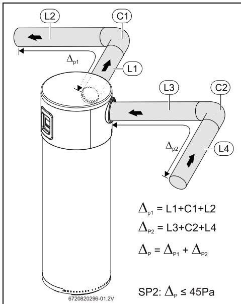
Bild 11 Äquivalente Leitungslänge (L)
