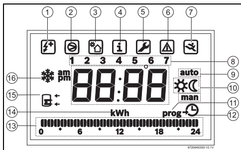
Bild 15 Display
