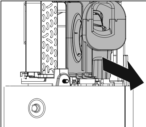
Bild 54 Baugruppe Luftführung und Gebläse entfernen
