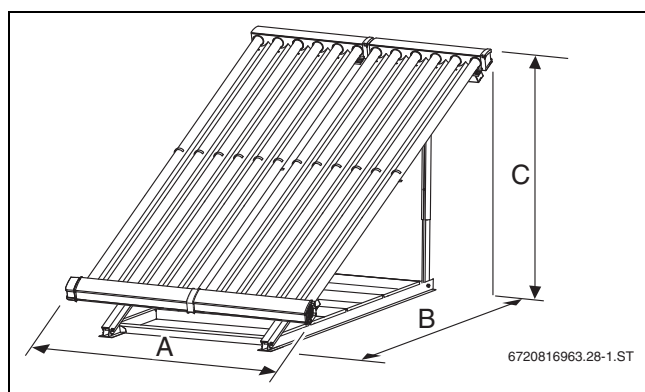
Bild 24 Maße Kollektorfeld
