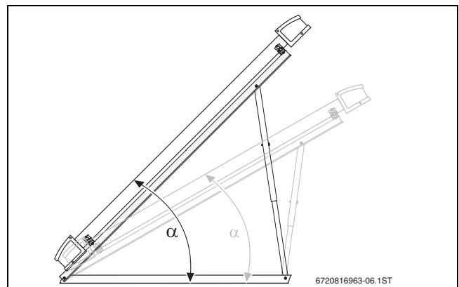
Bild 18 Anstellwinkel der Kollektoren
