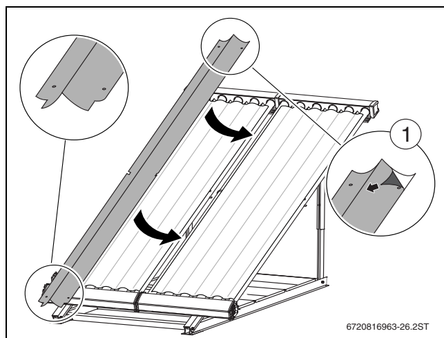
Bild 57 Zwischenspiegel einlegen
