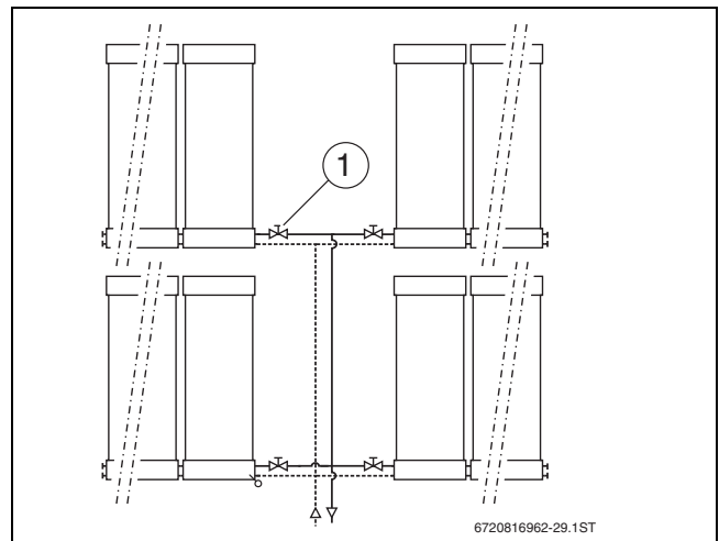
Bild 17 Maximal 7 Kollektoren je Einzelfeld (Parallelschaltung)
