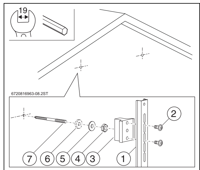
Bild 36 Profilschienen mit dem Stocksrauben-Set montieren
