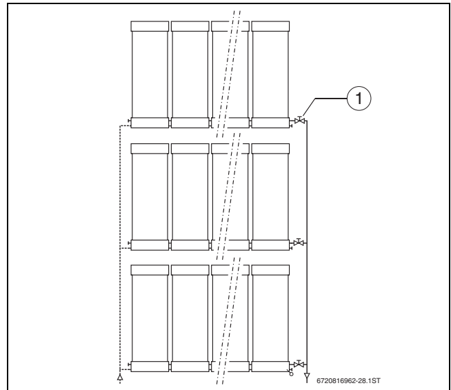
Bild 16 Maximal 14 Kollektoren je Reihe (Parallelschaltung)
