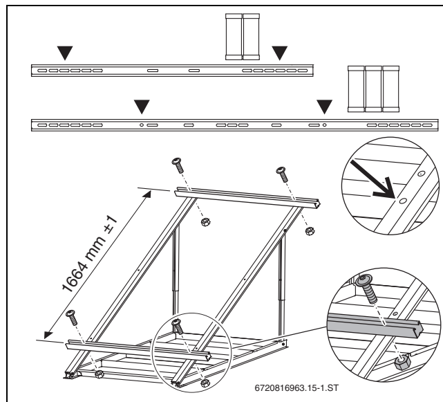
Bild 41 Profilschienen für 2 und 3 Kollektoren montieren
