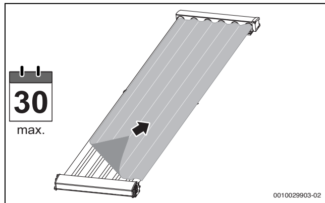
Bild 60 Kollektorfolie entfernen
