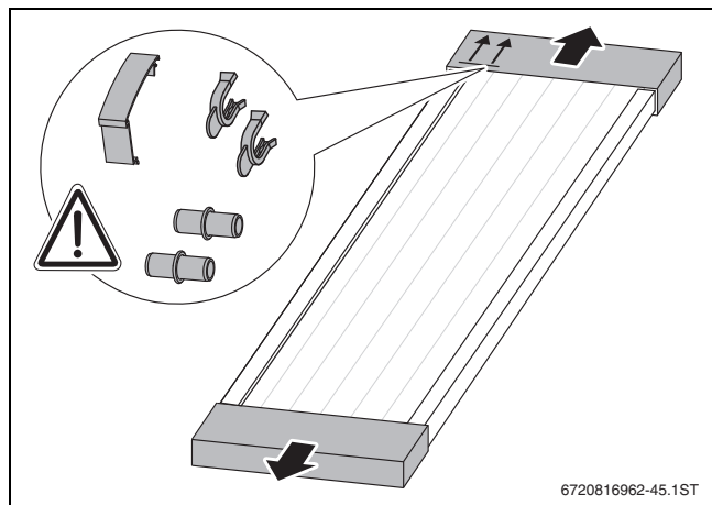
Bild 45 Verpackungsdeckel entfernen
