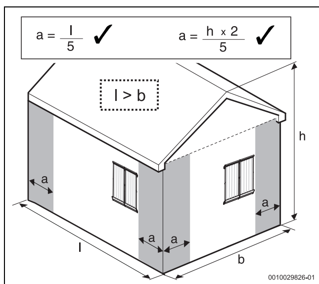
Bild 23 Einzuhaltende Abstandsmaße zum Gebäude [a]; der kleinere Wert kann genutzt werden
