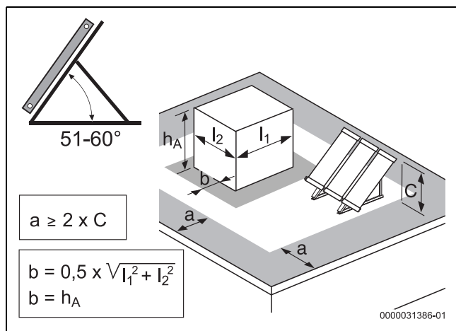
Bild 22 Bei Maß a ist der größere Wert maßgebend; bei [b] ist der kleinere Wert maßgebend (Anstellwinkel Kollektoren 51°-60°)
