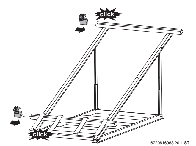
Bild 44 Kollektorspanner montieren
