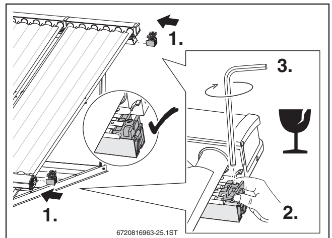
Bild 53 Kollektorspanner montieren
