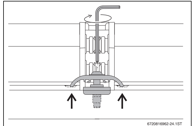
Bild 52 Doppelseitigen Kollektorspanner befestigen
