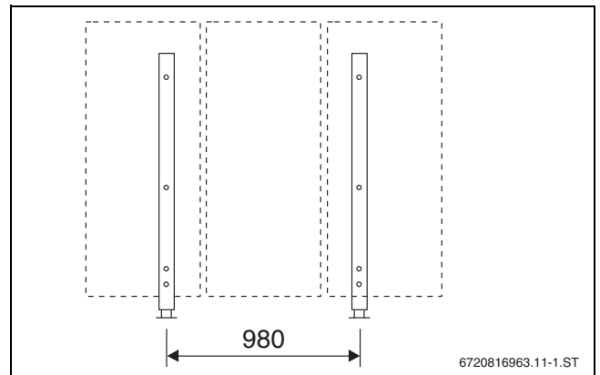
Bild 28 Grundauführung, 3 Kollektoren (Maße in mm)
