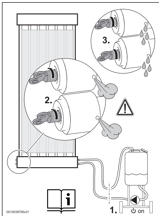
Bild 57 Entlüften
