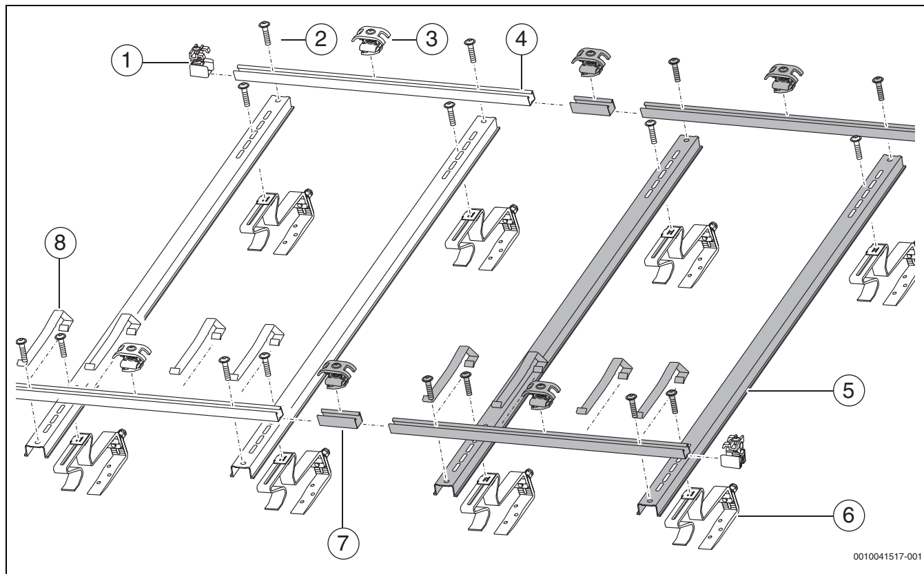
Bild 3 Montage-Set für 4 Kollektoren (grau: Montage-Set Erweiterung für 2 Kollektoren)
