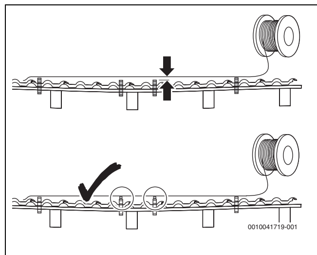
Bild 34 Einheitliche Höhe der Dachhaken prüfen
