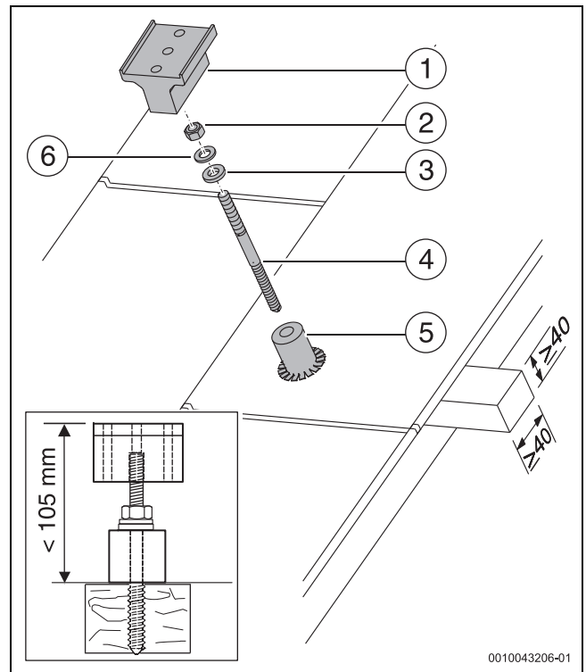
Bild 30 Stockschrabe montieren
