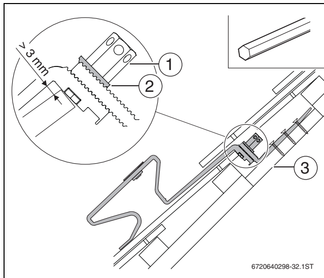
Bild 27 Sparrenanker montieren
