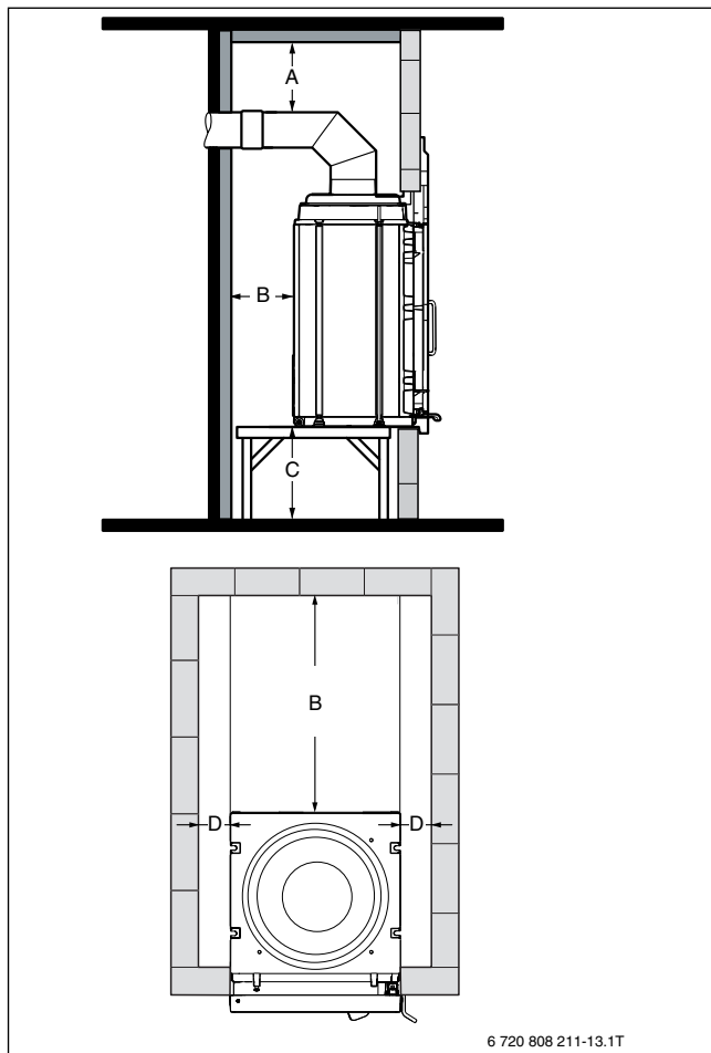
Bild 7 Heizkammer-Mindestabstände
