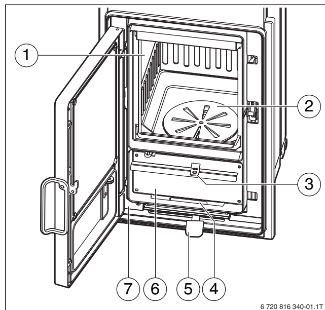
Bild 4 Heizeinsatz Rost
