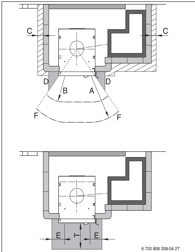
Bild 6 Heizkammer-Mindestabstände
