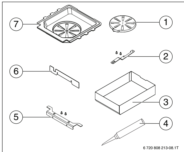
Bild 2 Lieferumfang – Rosteinsatz
