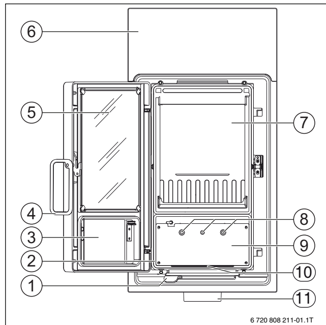
Bild 3 Heizeinsatz Mulde
