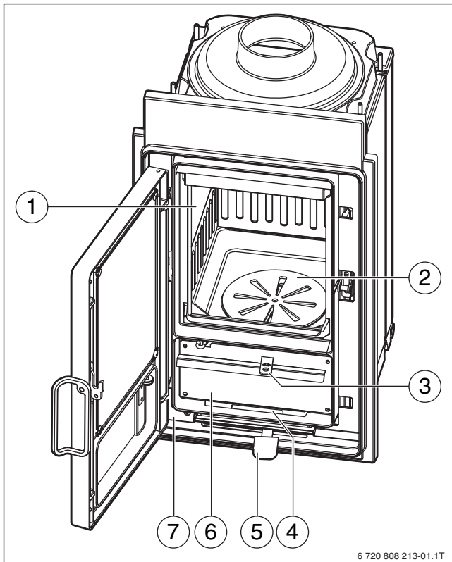
Bild 2 Heizeinsatz Rost
