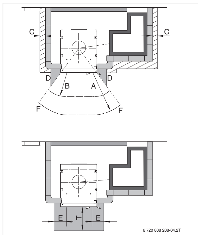
Bild 4 Äußere Mindestabstände
