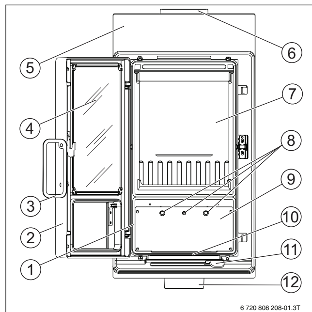
Bild 1 Heizeinsatz Mulde
