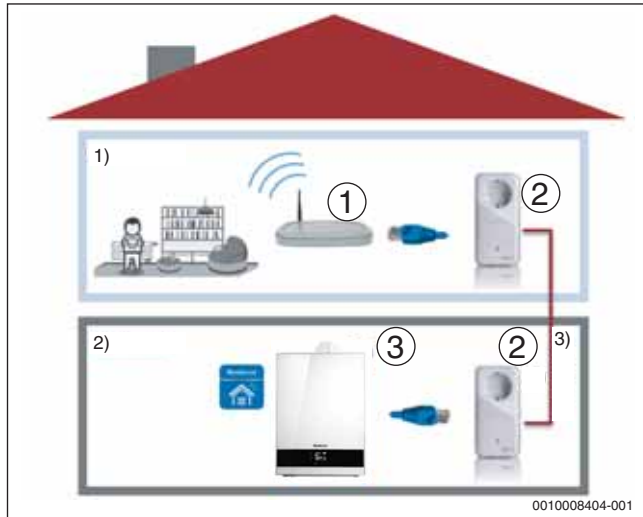
Bild 3 PowerLAN
