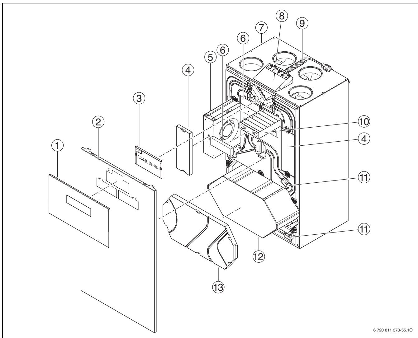
Bild 5 Wohnungslüftungsgerät Logavent HRV2-140 (S)
