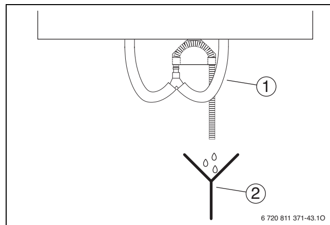
Bild 25 Kondensatableitung
