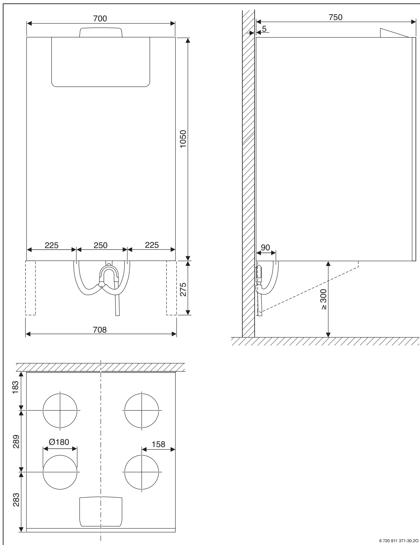
Bild 4 Logavent HRV2-350 (S)
