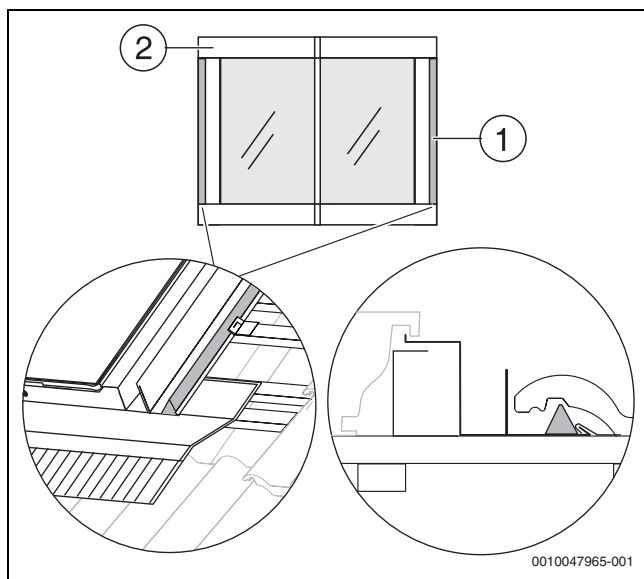
Bild 77 Dreieckdichtband einlegen
