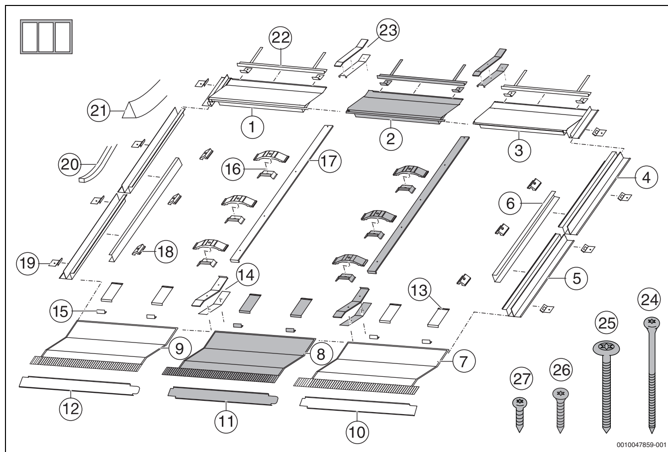
Bild 4 Montage-Set für 3 senkrechte Kollektoren: 1 × Grundaufbau für die ersten beiden Kollektoren und 1 × Montage-Set Erweiterung (grau) für jeden weiteren Kollektor
