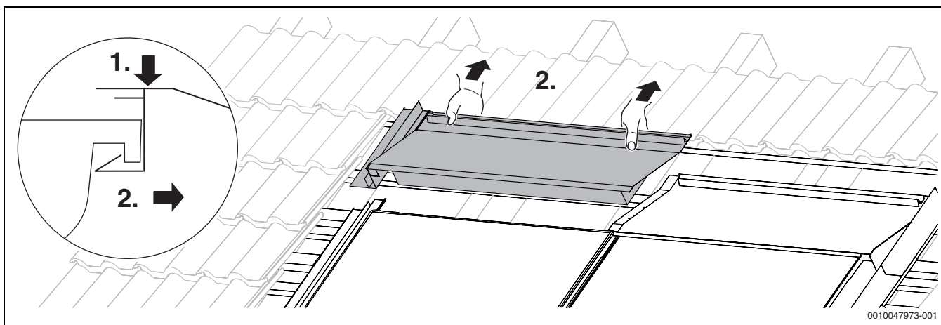
Bild 86 Eindeckblech abziehen
