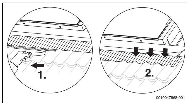
Bild 80 Bleischürzen auf Eindeckung kleben
