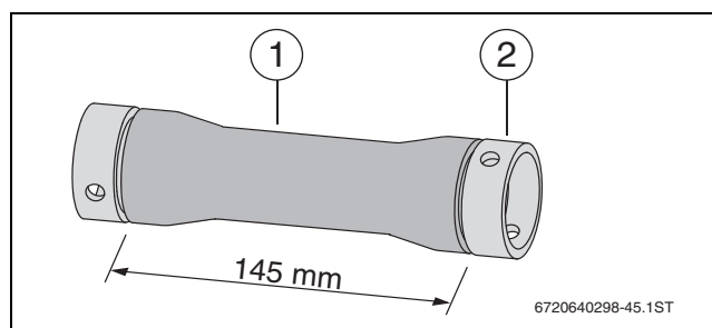
Bild 16 Solarschlauch mit Stopfen
