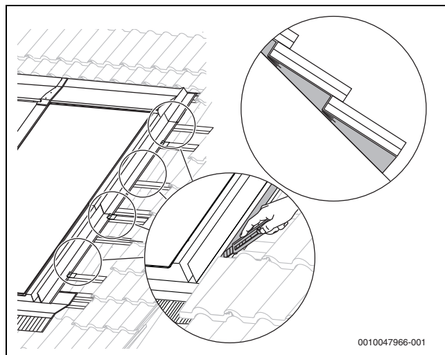
Bild 78 Dreieckdichtband einschneiden
