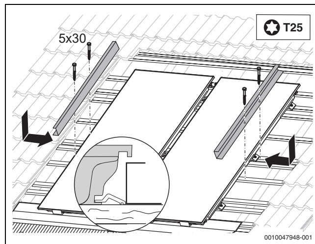
Bild 61 Seitliche Stützbleche montieren
