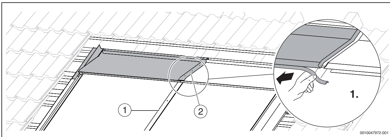
Bild 85 Dichtlippe abziehen
