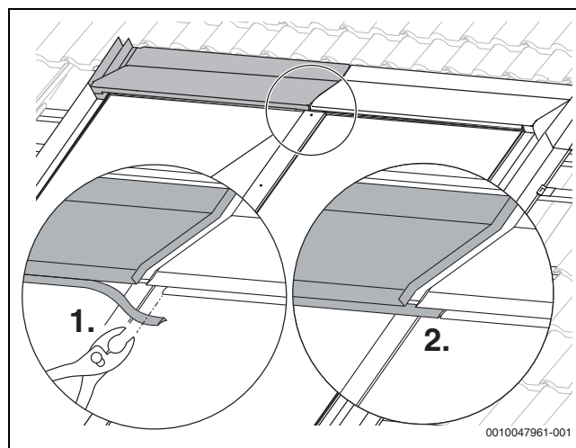
Bild 74 Dichtlippe anpassen
