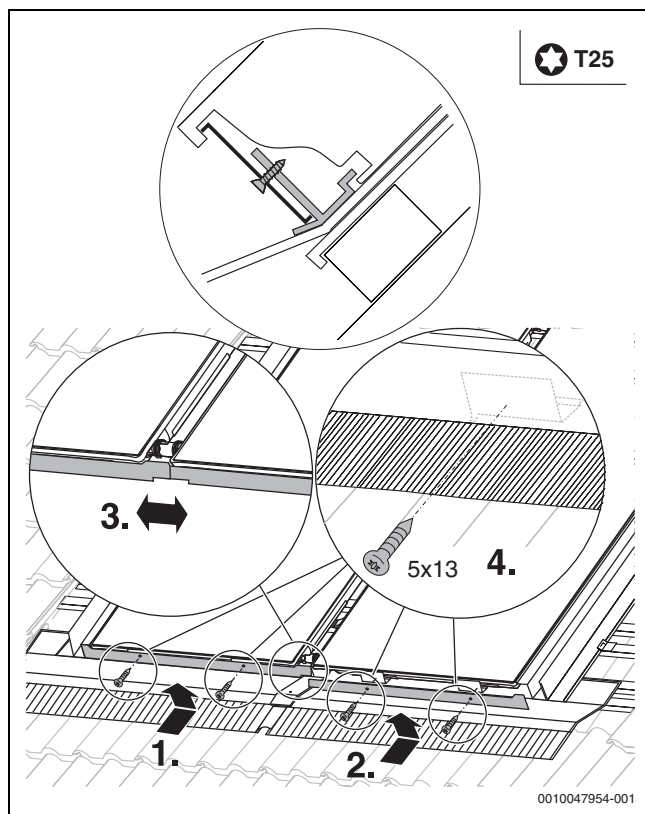
Bild 67 Blenden festschrauben
