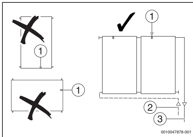
Bild 11 Kollektoranordnung
