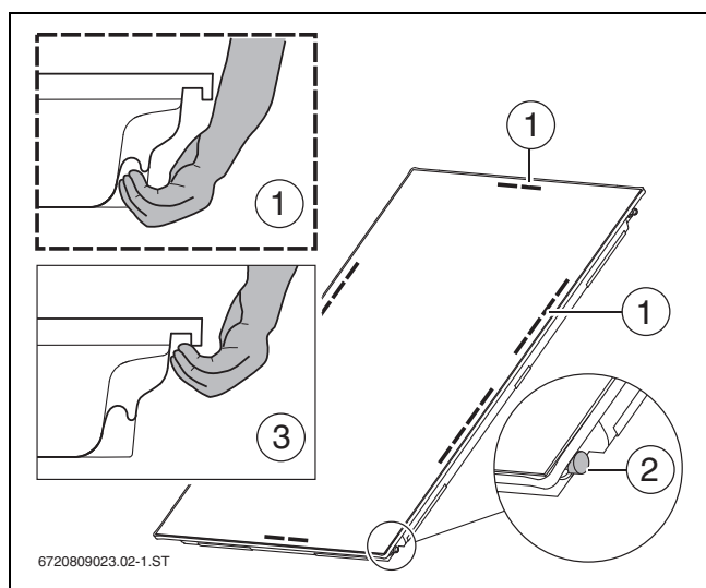
Bild 15 Kollektor tragen
