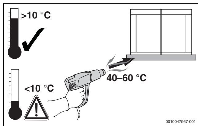
Bild 79 Bleischürze erwärmen, wenn erforderlich
