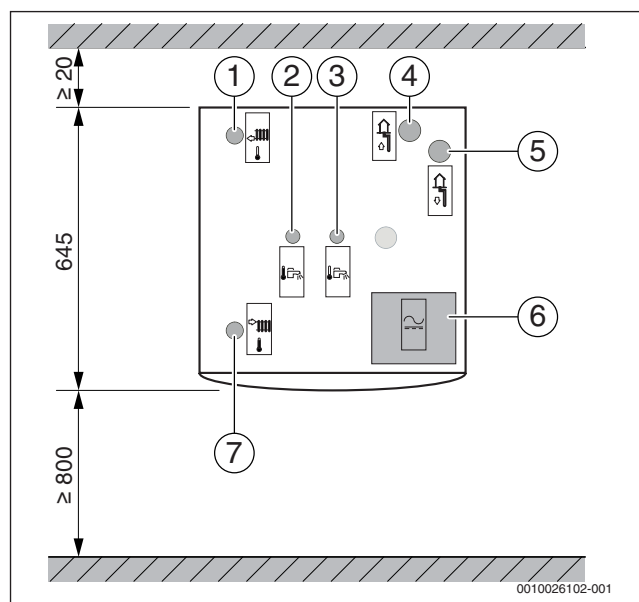
Bild 5 Abmessungen und Mindestabstände WPS ..K-1 (Draufsicht)
