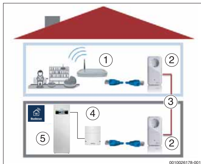
Bild 15 PowerLAN
