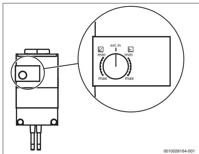
Bild 10 Einstellungen an der primären Heizkreispumpe
