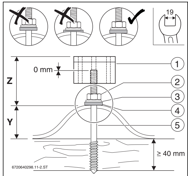
Bild 26 Montierte Stockschraube mit Haltebock
