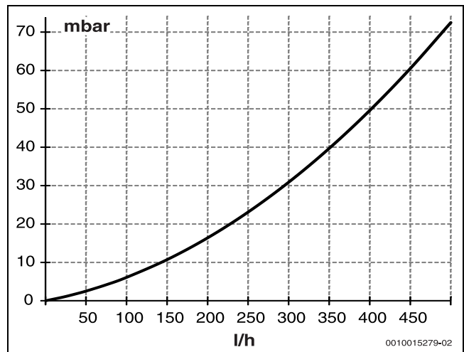
Bild 2 Druckverlustkurve
