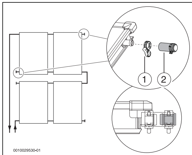
Bild 55 Stopfen montieren
