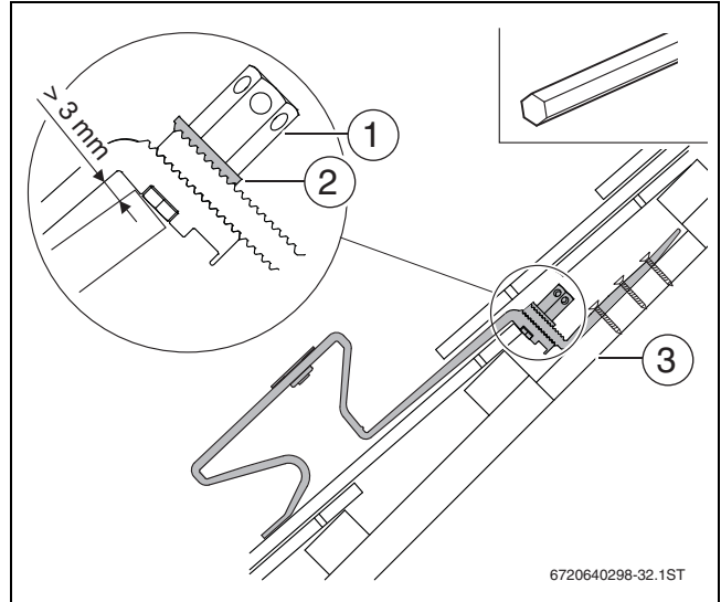
Bild 20 Sparrenanker montieren
