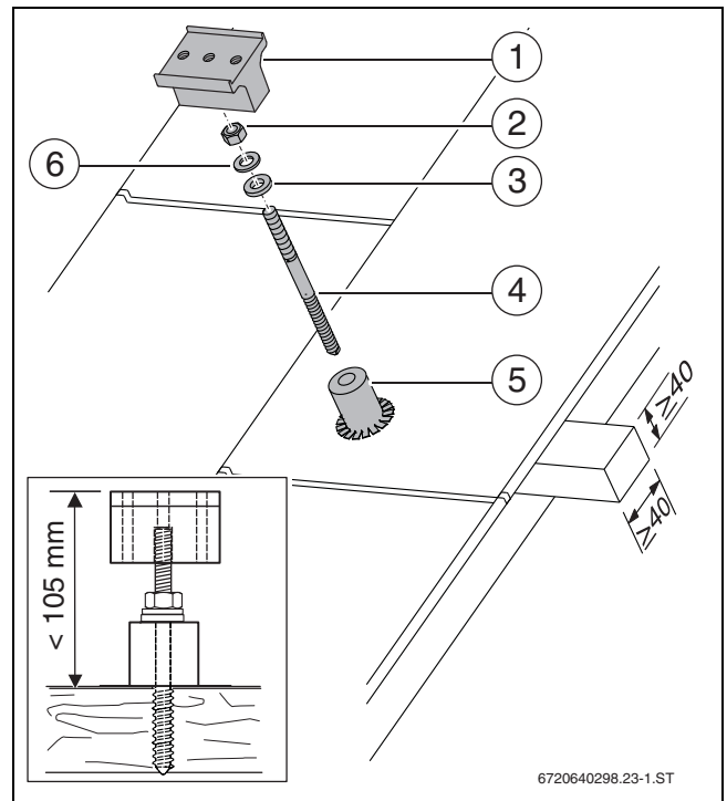
Bild 23 Stockschraube montieren
