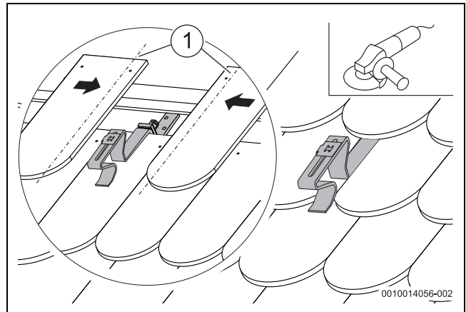
Bild 21 Biberschwanzziegel anpassen
