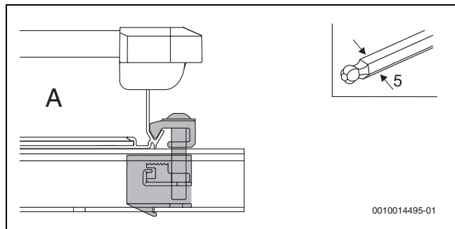
Bild 39 Kollektorspanner festdrehen
