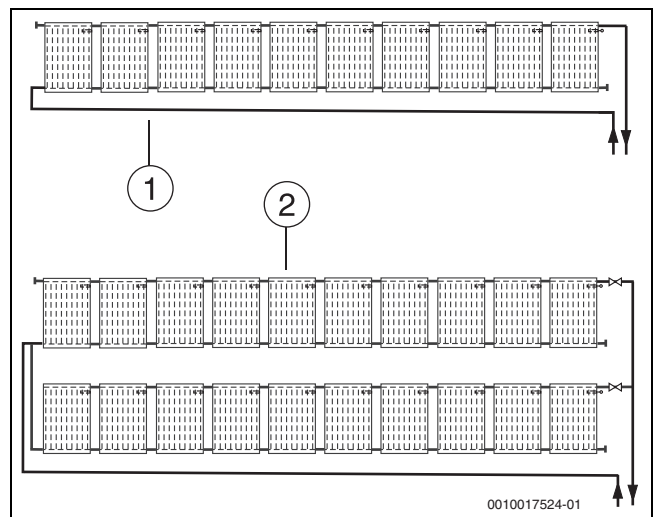
Bild 10 Hydraulischer Anschluss
