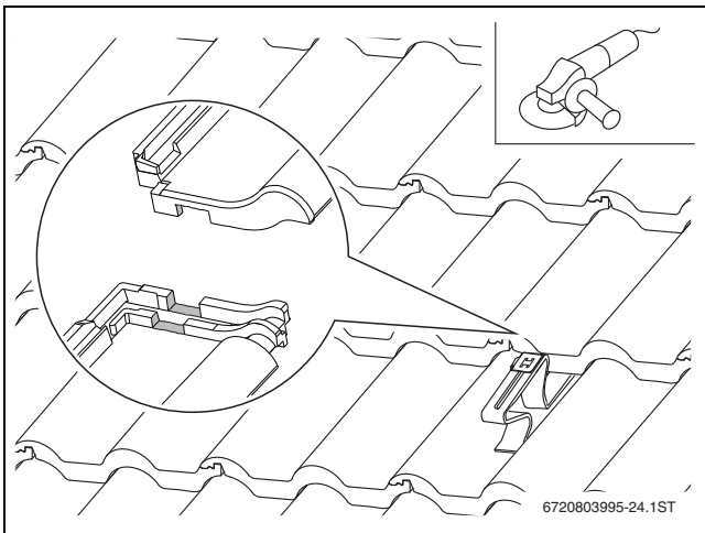
Bild 16 Dachziegel anpassen
