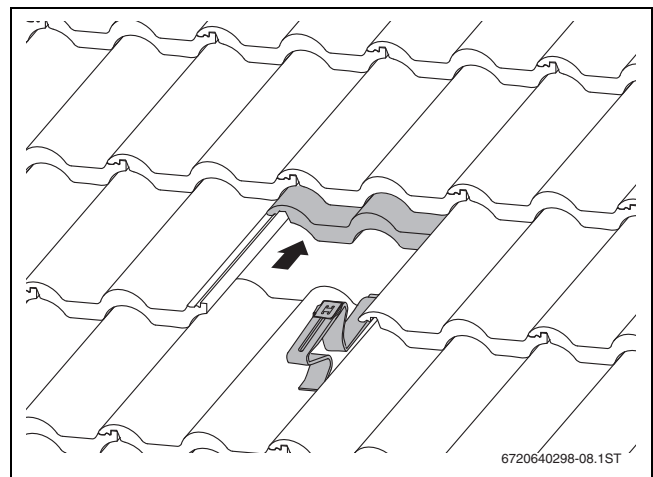
Bild 14 Eingängter Dachhaken
