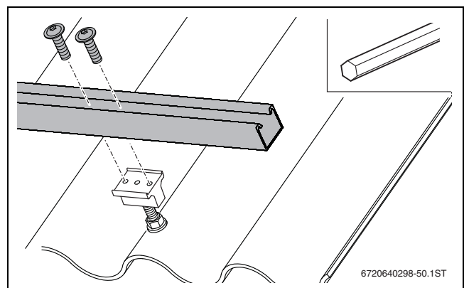
Bild 27 Profilschienen montieren
