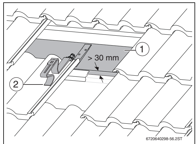
Bild 18 Sparrenanker auf Brett/Bohle montieren
