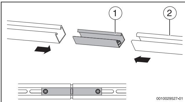
Bild 29 Profilschienen verbinden
