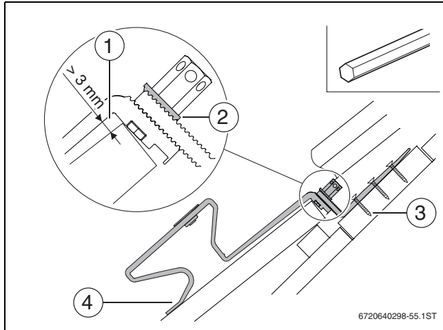
Bild 19 Sparrenanker befestigen
