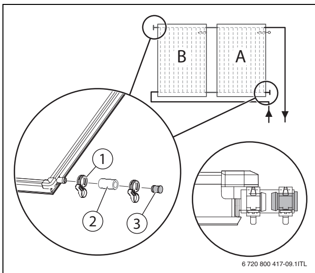
Bild 35 Stopfen montieren
