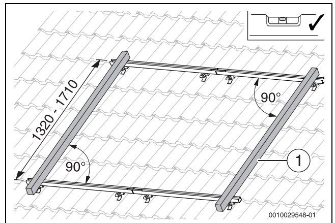
Bild 31 Profilschienen ausrichten
