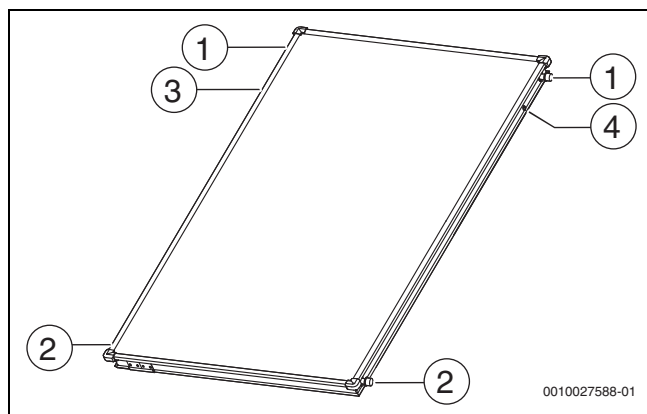
Bild 1 Kollekortyp senkrecht
