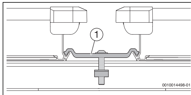
Bild 42 Doppelseitiger Kollektorspanner
