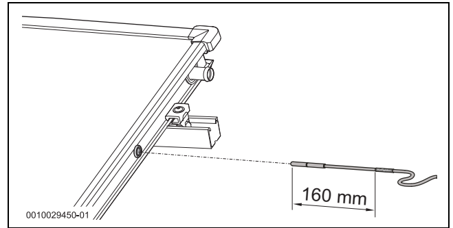
Bild 46 Kollektortemperaturfühler montieren
