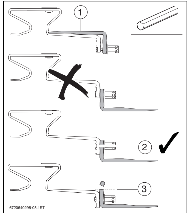
Bild 17 Sparrenanker vorbereiten
