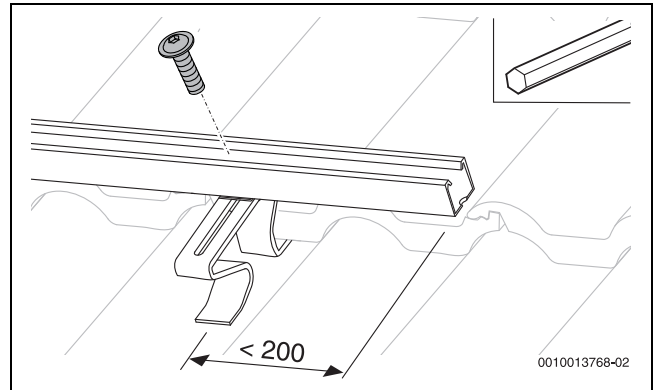
Bild 30 Profilschiene montieren
