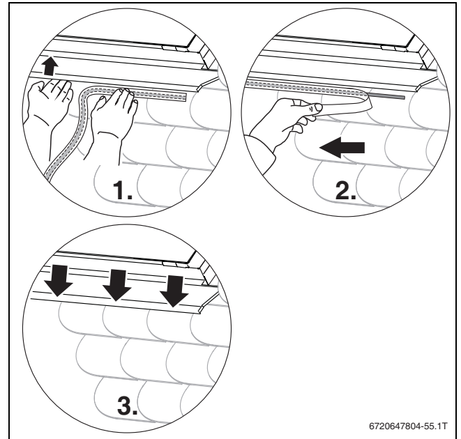
Bild 78 Unterer Eindeckblech auf Eindeckung kleben
