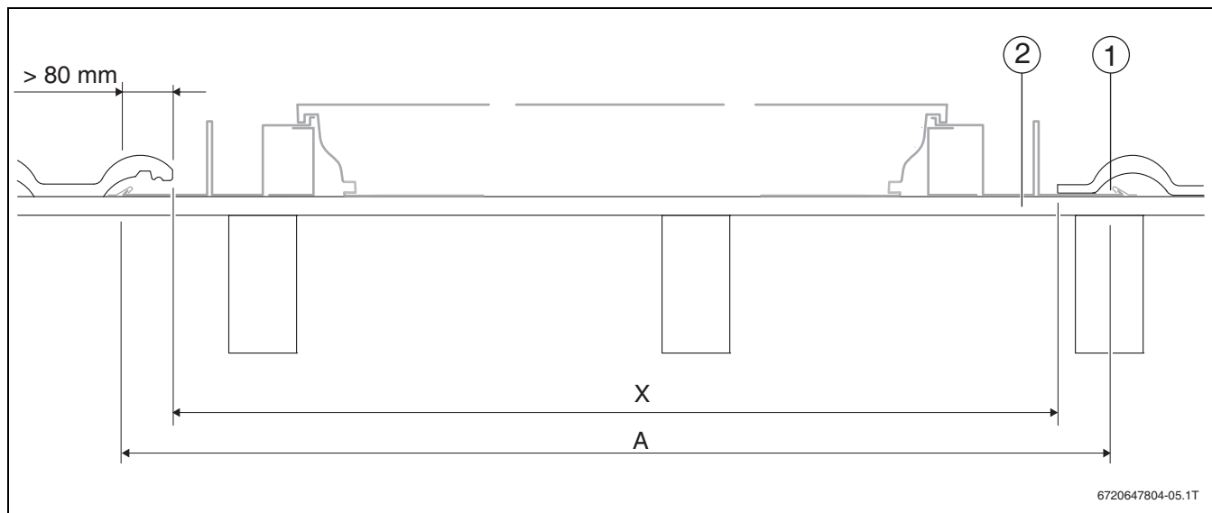
Bild 23 Kollektorfeldbreite
