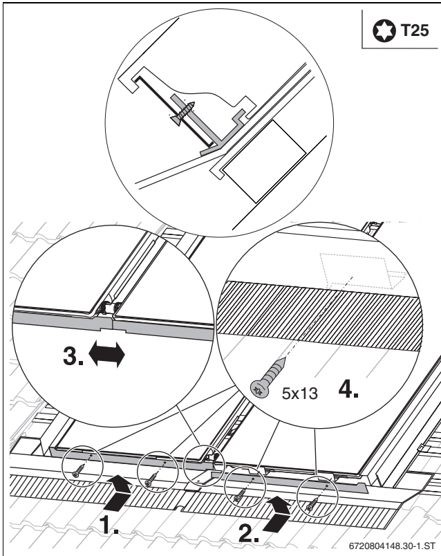
Bild 65 Blenden festschrauben
