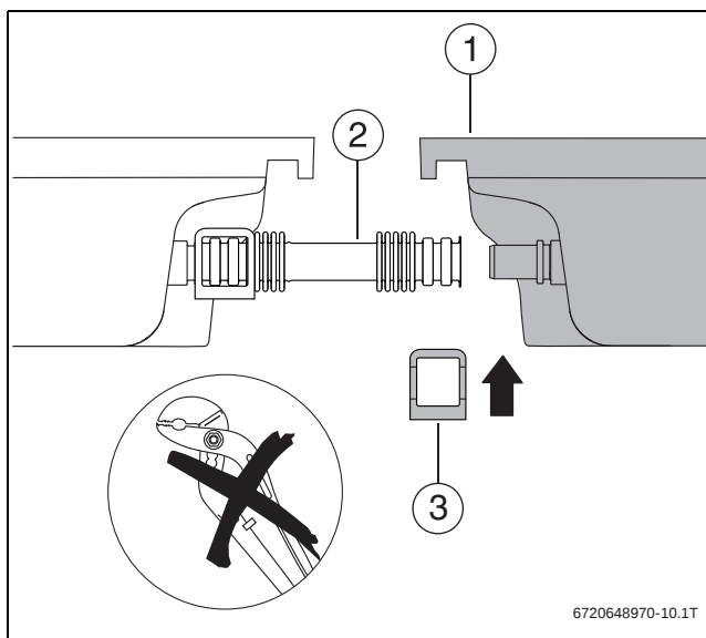
Bild 47 Wellrohrverbinder sichern
