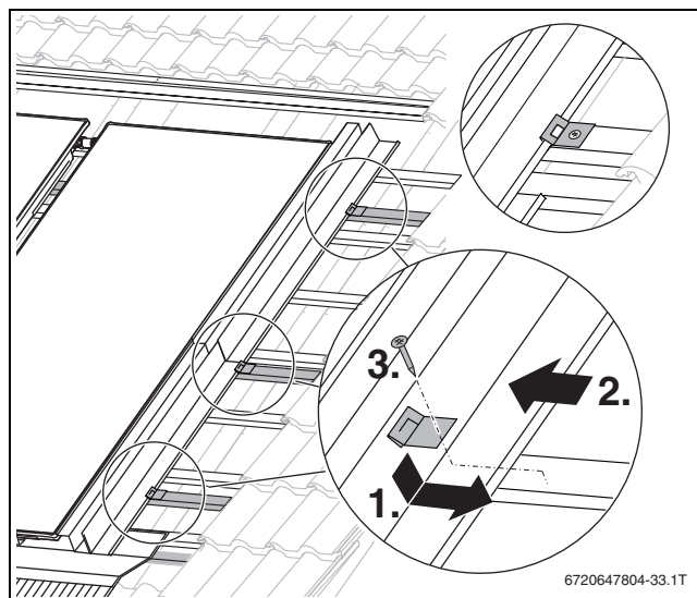
Bild 63 Hafter montieren
