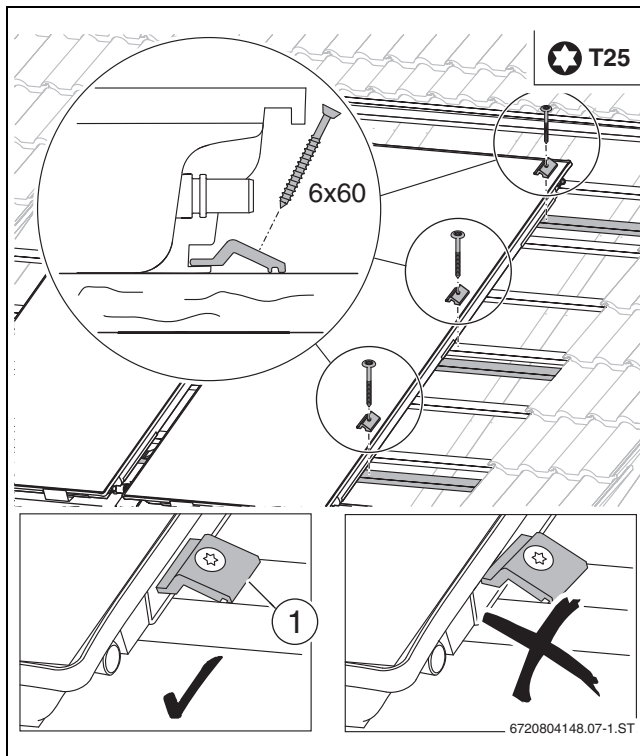
Bild 51 Niederhalter festschrauben
