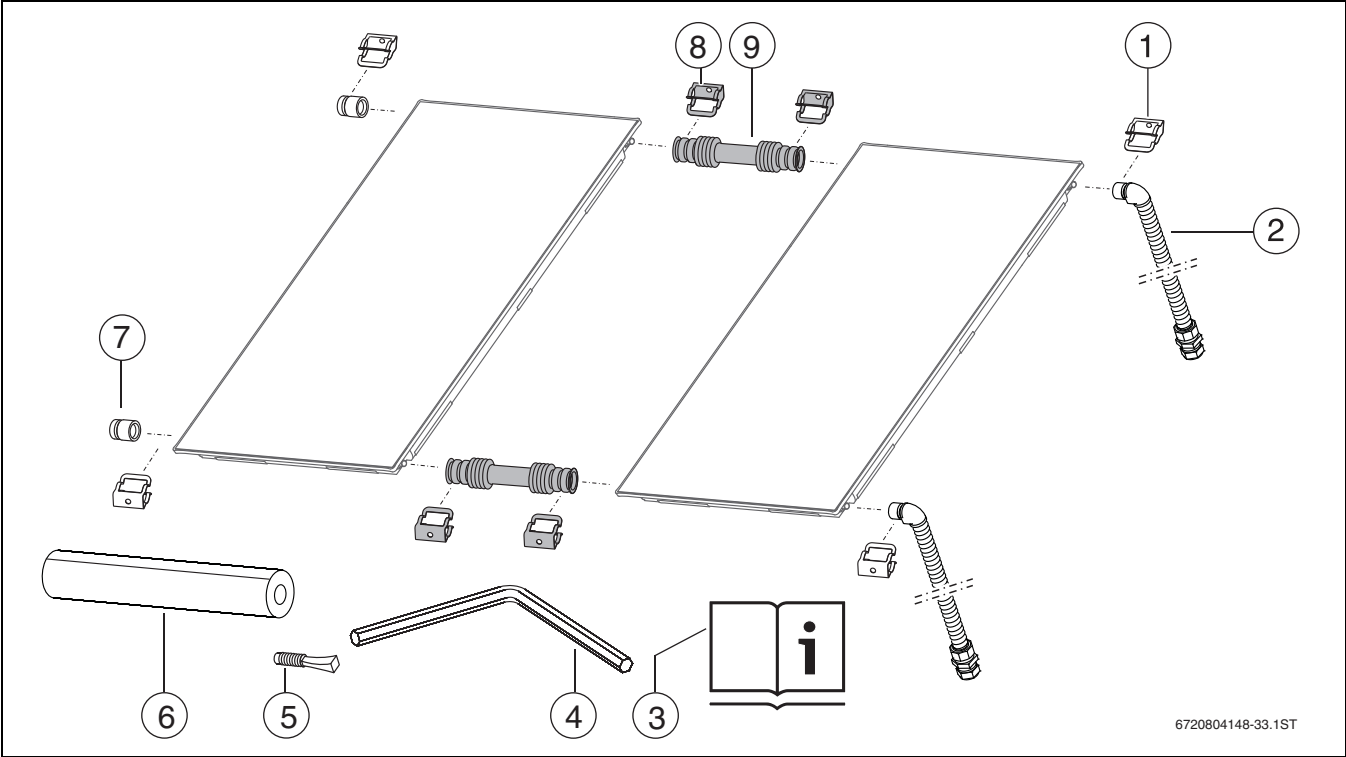
Bild 8 1 Anschluss-Set Indach und 2 Verbindungs-Sets (grau)
