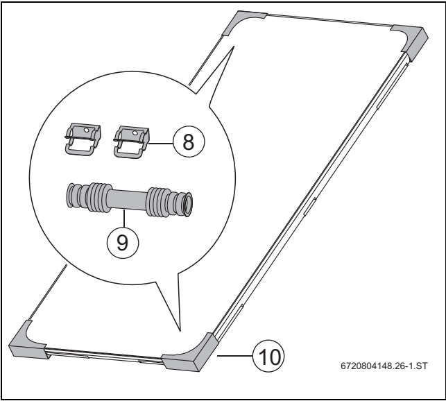
Bild 9 2 Transportschutzecken beinhalten je 1 Verbindungs-Set (1 Verbindungs-Set enthält 2 Klammern und 1 Wellrohrverbinder)
