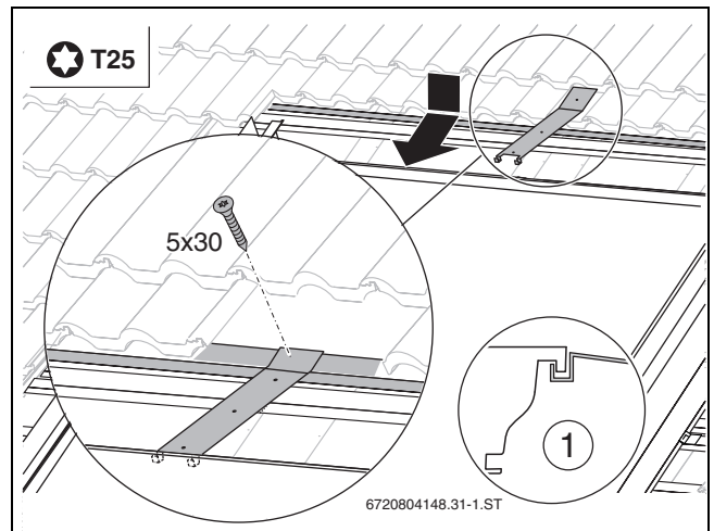
Bild 68 Waagerechte Ausführung
