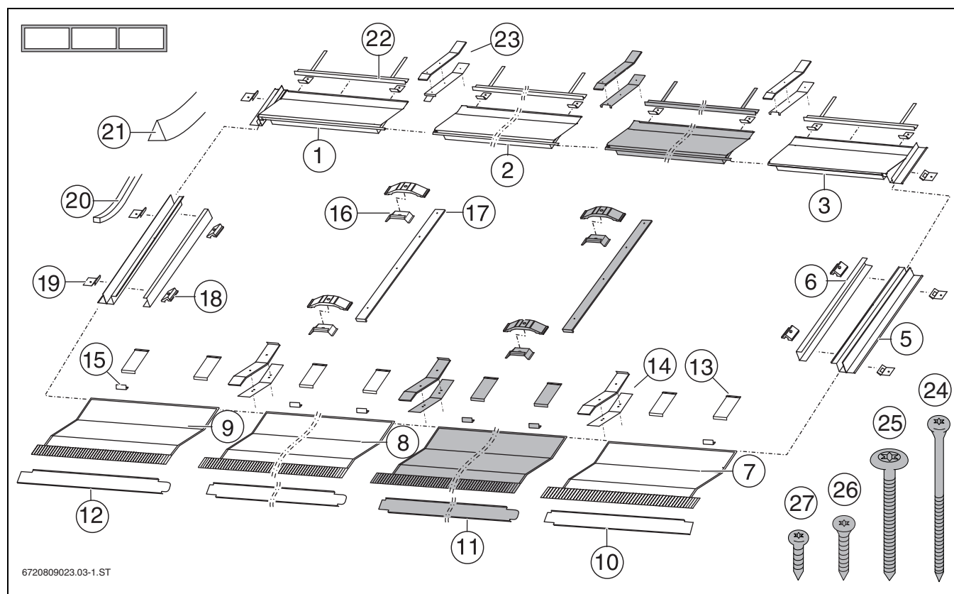
Bild 6 Montage-Set für 3 waagerechte Kollektoren: 1 Montage-Set Grundauführung für die ersten beiden Kollektoren und 1 x Montage-Set Erweiterung (grau) für jeden weiteren Kollektor
