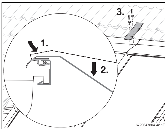
Bild 73 Oberteil des Verbinders montieren
