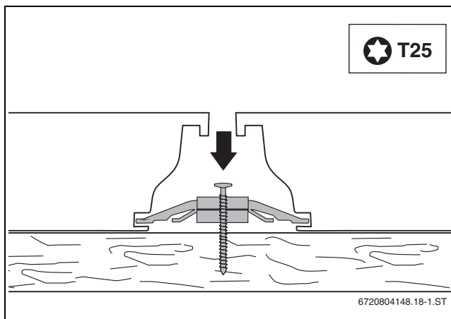
Bild 49 Schrauben festziehen
