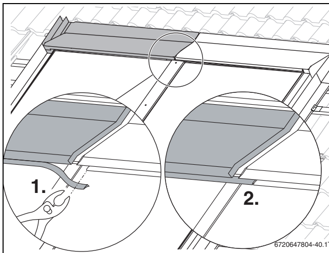
Bild 71 Dichtlippe anpassen
