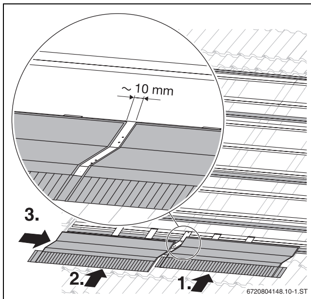
Bild 32 Eindeckbleche für 2 Kollektoren
