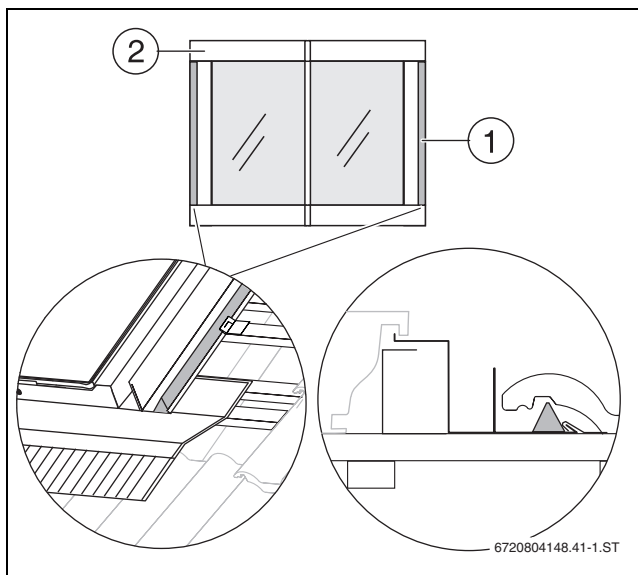
Bild 74 Dreiecksdichtband einlegen
