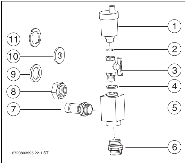
Bild 57 Lieferumfang Entlüfter-Set
