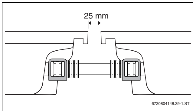
Bild 48 Gesicherter Wellrohrverbinder
