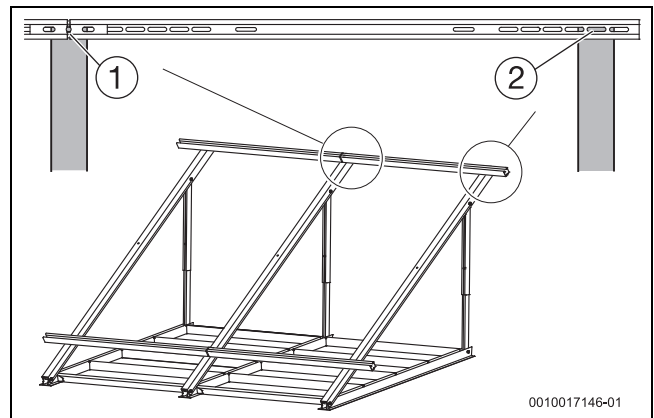
Bild 44 Profilschienen positionieren
