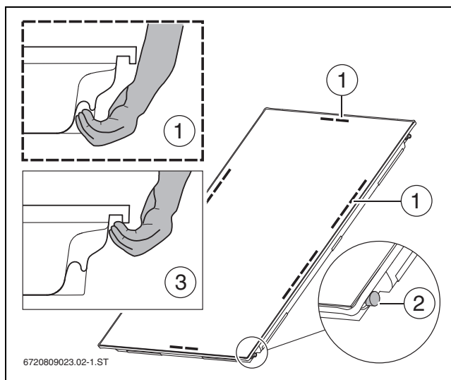
Bild 25 Kollektor tragen
