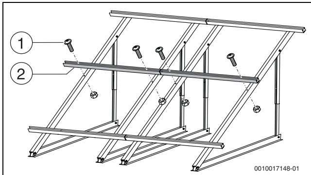
Bild 46 Zusätzliche Profilschienen montieren (hier: 2 Kollektoren)
