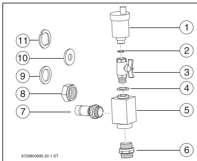
Bild 64 Lieferumfang Entlüfter-Set
