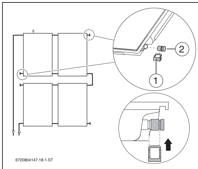
Bild 66 Kappen montieren
