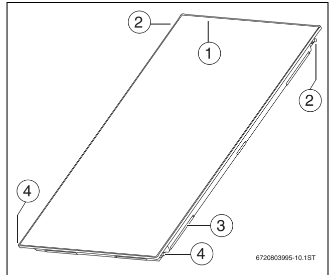
Bild 1 Kollektortyp senkrecht
