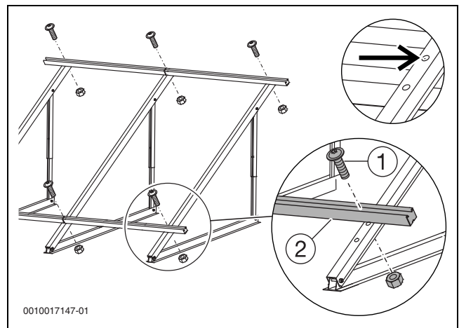
Bild 45 Profilschienen montieren
