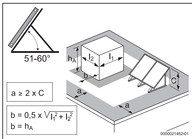
Bild 22 Bei Maß [a] ist der größere Wert maßgebend; bei [b] ist der kleinere Wert maßgebend; Anstellwinkel Kollektoren 51-60° (absoluter Winkel zur Horizontalen)
