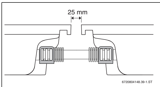
Bild 57 Kollektoren zusammengeschoben
