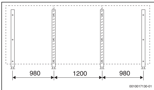
Bild 31 Grundauführung, 3 senkrechte Kollektoren (Maße in mm)
