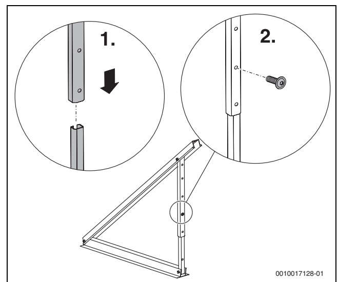
Bild 29 Teleskopschienen montieren
