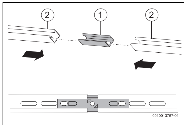
Bild 43 Profilschienen verbinden
