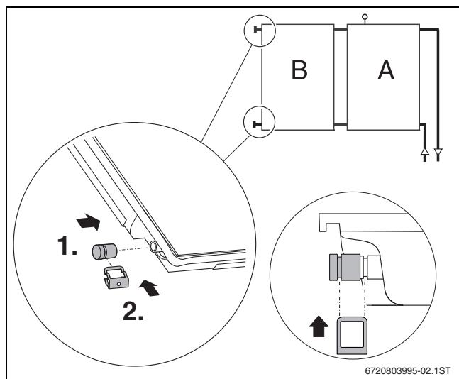
Bild 49 Kappen montieren
