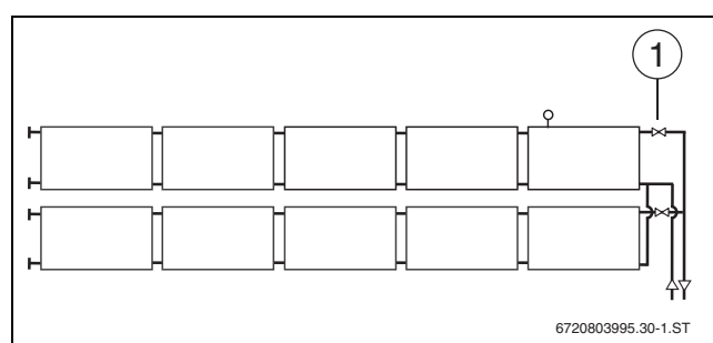
Bild 15 Gleichseitiger Anschluss einer Parallelschaltung
