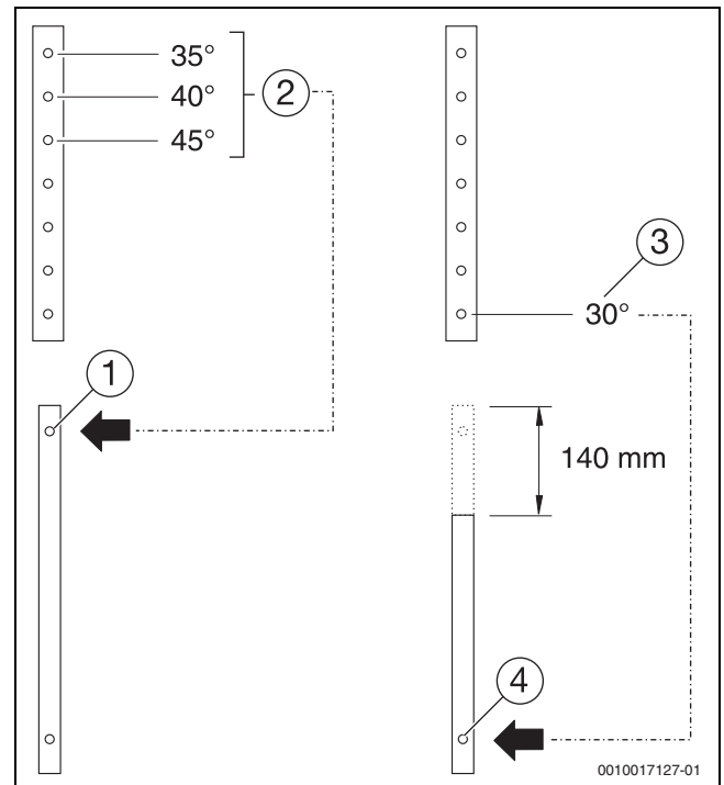
Bild 28 Teleskopschienen montieren - Kollektortyp waagrecht
