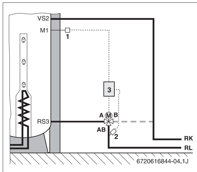
Bild 6 Montageschema Pufferspeicher
