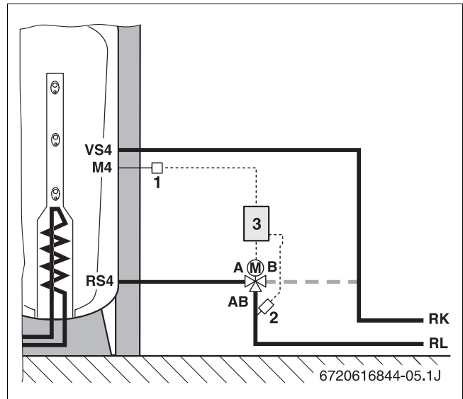
Bild 7 Montageschema Kombispeicher
