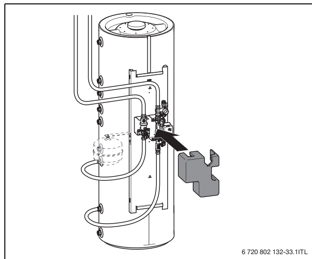
Bild 25 Isolierhaube aufsetzen
