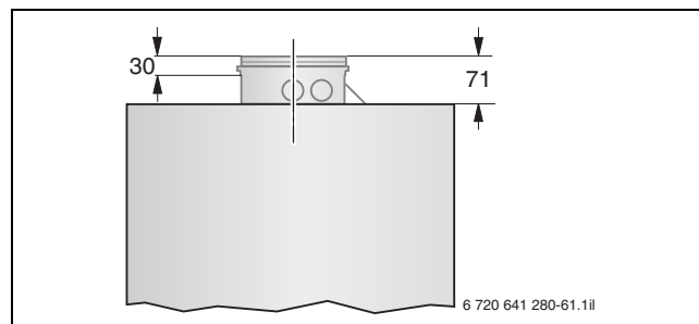
Bild 121 Montage Maße des konzentrischen Anschlussstücks (Maße in mm)
