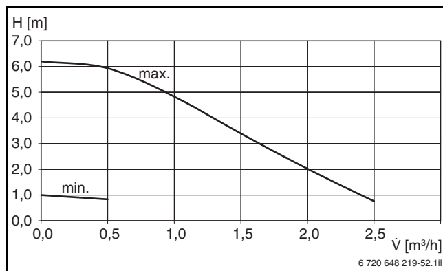
Bild 94 Restförderhöhe HSM 25-E plus
