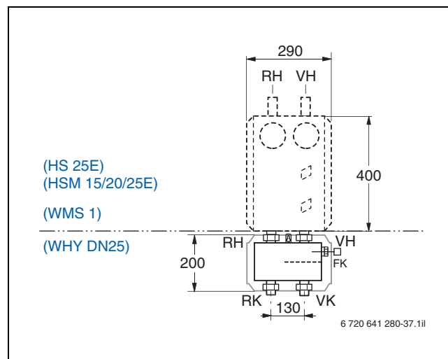
Bild 87 Abmessungen der Systemkombination mit hydraulischer Weiche quer zur direkten Verbindung mit einem Heizkreis-Anschluss-Set für einen Heizkreis (Maße in mm)
