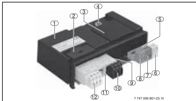
Bild 46 Weichenmodule WM10 (Basismodul)
