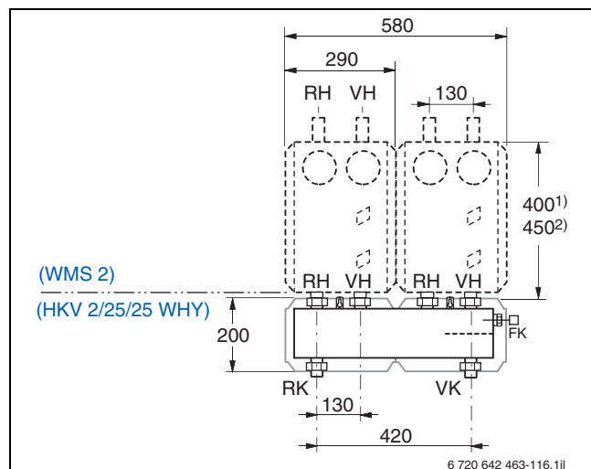
Bild 86 Abmessungen der Systemkombination Heizkreisverteiler mit integrierter hydraulischer Weiche für zwei Heizkreise (Maße in mm)
