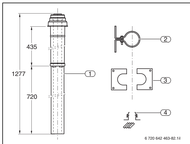
Bild 122 Bauteile des Grundbausatzes DO aus Kunststoff (Maße in mm)
