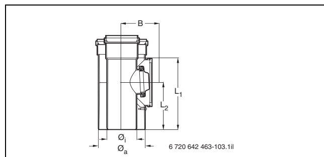
Bild 156 Konzentrisches Rohr mit Prüföffnung Ø 80/125
