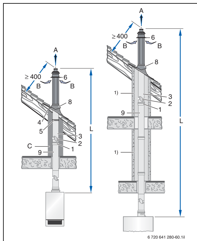
Bild 120 Montagevarianten (Maße in mm)
