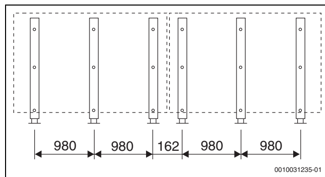
Bild 32 Ausführung für höhere Lasten, 2 waagerechte Kollektoren, Anstellwinkel 30-35°
