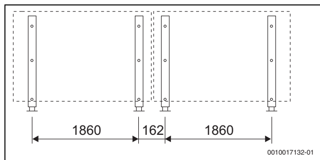
Bild 30 Grundausführung, 2 waagerechte Kollektoren (Maße in mm)
