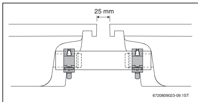
Bild 56 Kollektoren zusammengeschoben
