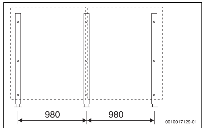
Bild 27 Grundaufführung, 2 senkrechte Kollektoren (Maße in mm)
