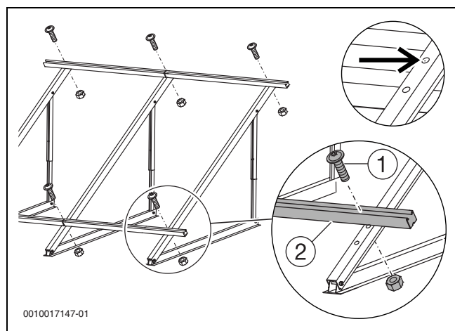
Bild 42 Profilschienen montieren
