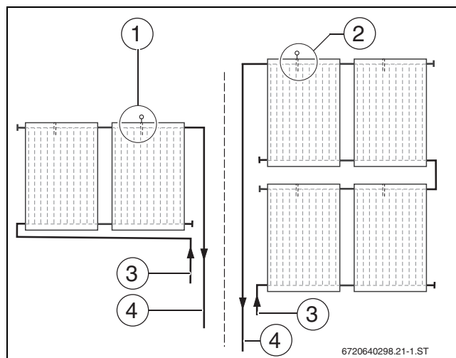
Bild 58 Position des Kolleortemperaturfühlers
