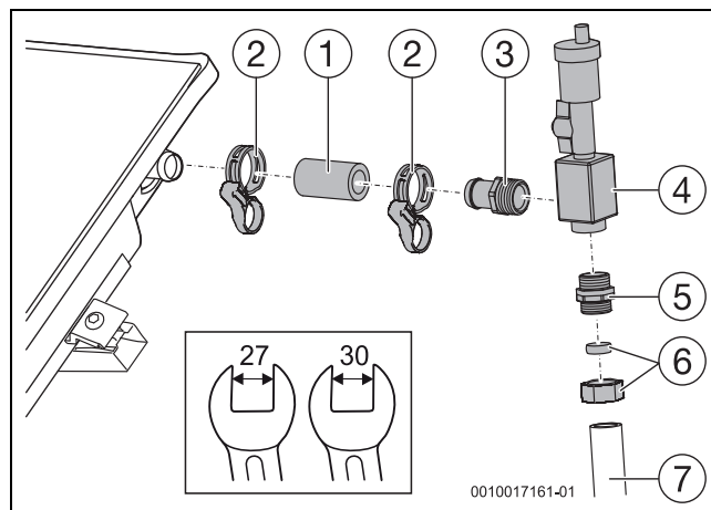
Bild 65 Vorlauf mit Entlüfter über Dach
