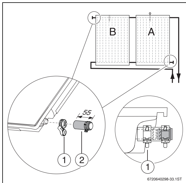
Bild 48 Stopfen montieren
