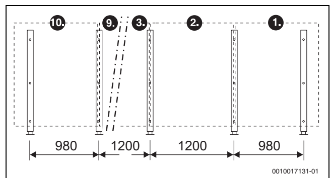
Bild 29 Grundaufführung, > 3 senkrechte Kollektoren (Maße in mm)
