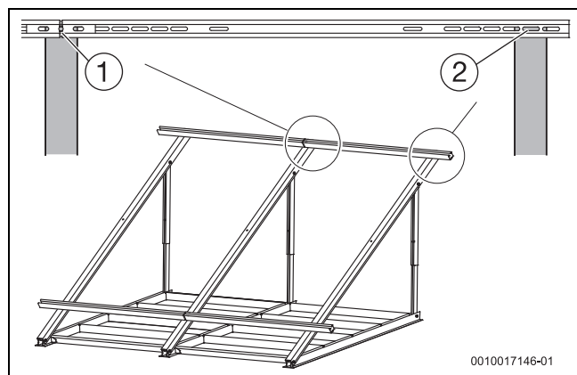
Bild 41 Profilschienen positionieren
