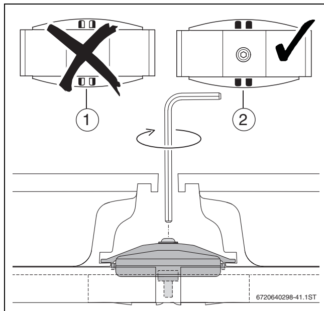
Bild 55 Kollektorspanner montiert
