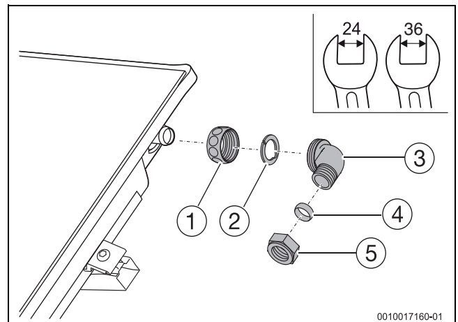
Bild 62 Winkeltülle montieren
