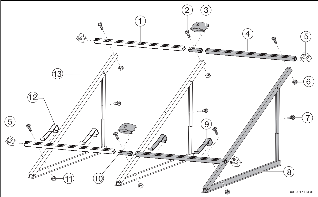
Bild 5 Montage-Set für 2 Kollektoren: 1 Montage-Set Grundaufführung, 1 Montage-Set Erweiterung (grau)
