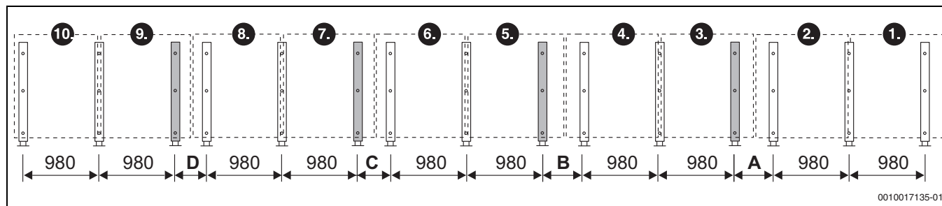
Bild 33 Grundausführung Beschwerungswannen, 10 senkrechte Kollektoren (Angaben in mm)
