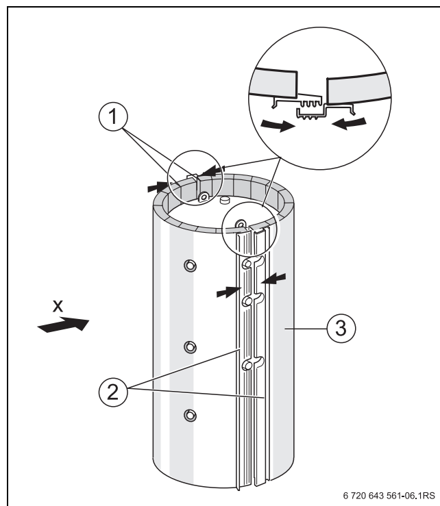
Bild 6 Wärmeschutz montieren
