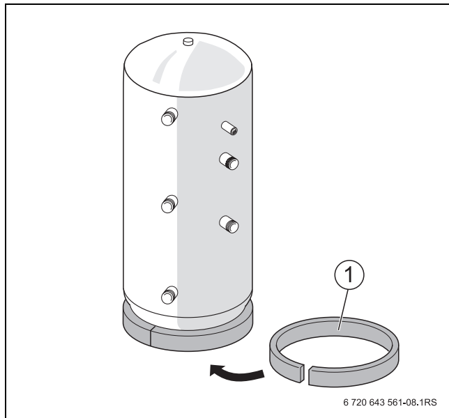
Bild 5 Unterer Wärmeschutzring
