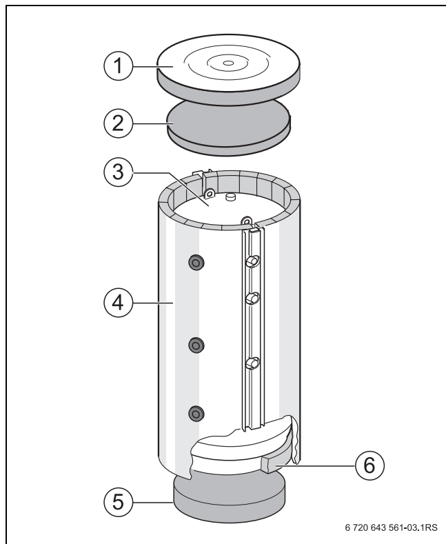
Bild 1 Pufferspeicher
