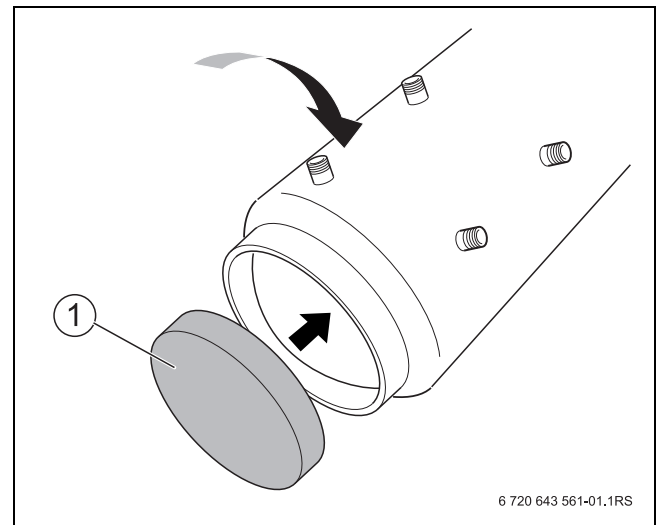
Bild 4 Untere Wärmeschutzscheibe einlegen
