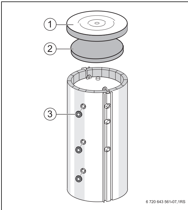
Bild 7 Speicherhaube montieren
