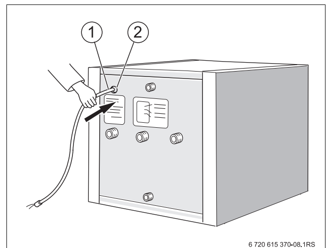
Bild 9 Warmwasser-Temperaturfühler montieren
