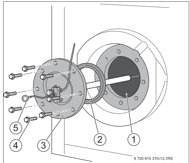
Bild 16 Inspektionsöffnung schließen
