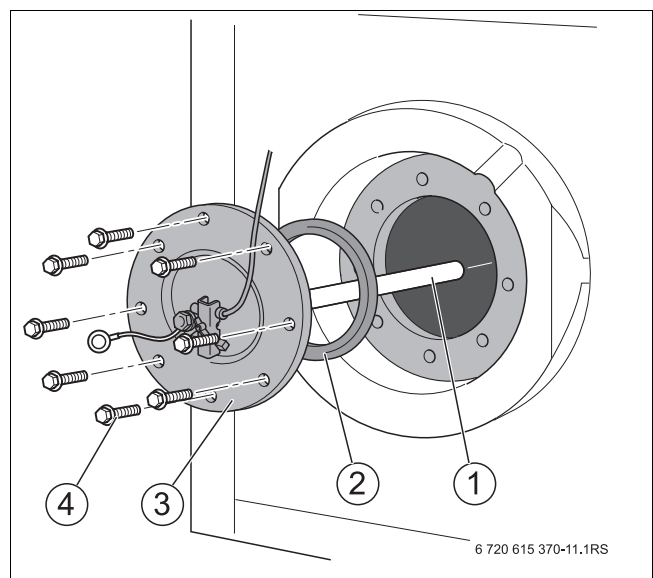
Bild 13 Inspektionsöffnung öffnen
