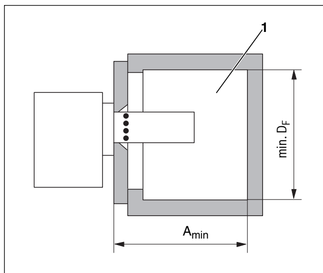
Bild 6 Feuerraum
