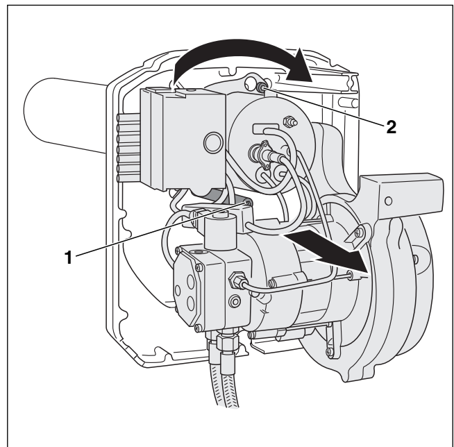
Bild 18 Brennergehäuse demontieren
