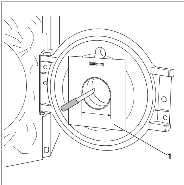
Bild 16 Türdämmung ausschneiden
