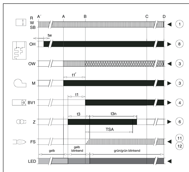
Bild 15 Programmablauf Ölfeuerungsautomat
