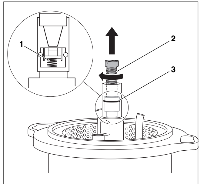
Bild 50 Abschlussventil austauschen
