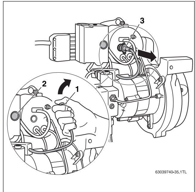
Bild 57 Flammenfühler auf Funktion prüfen
