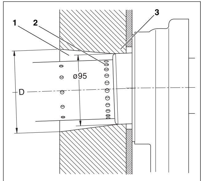
Bild 17 Schnittzeichnung des Türausschnitts (Maß in mm)
