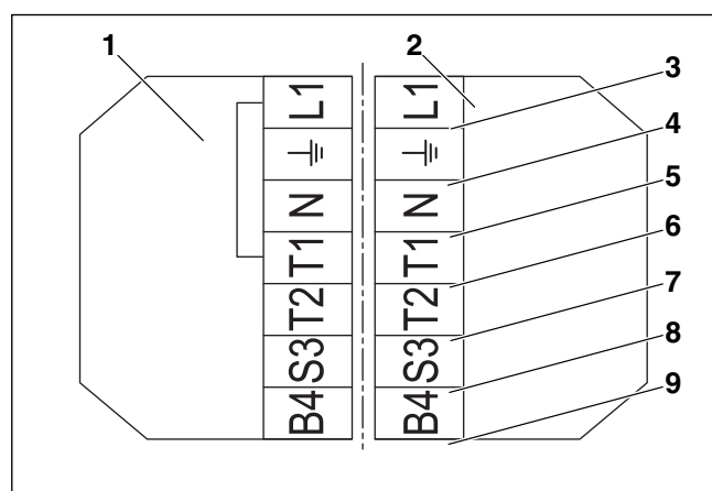
Bild 13 Brenneranschlussleitung – 7-poliger-Brennerstecker
