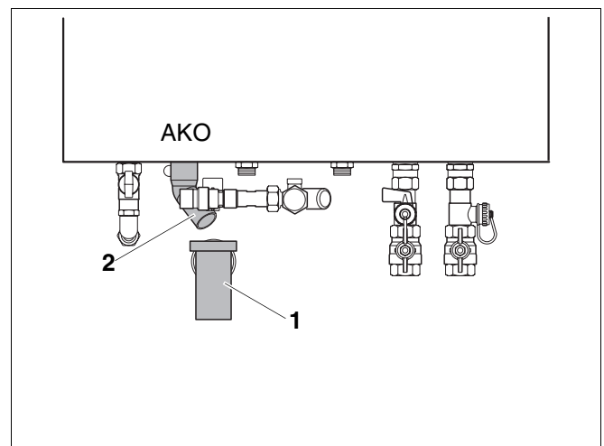
Abb. 10 Trichtersiphon montieren
