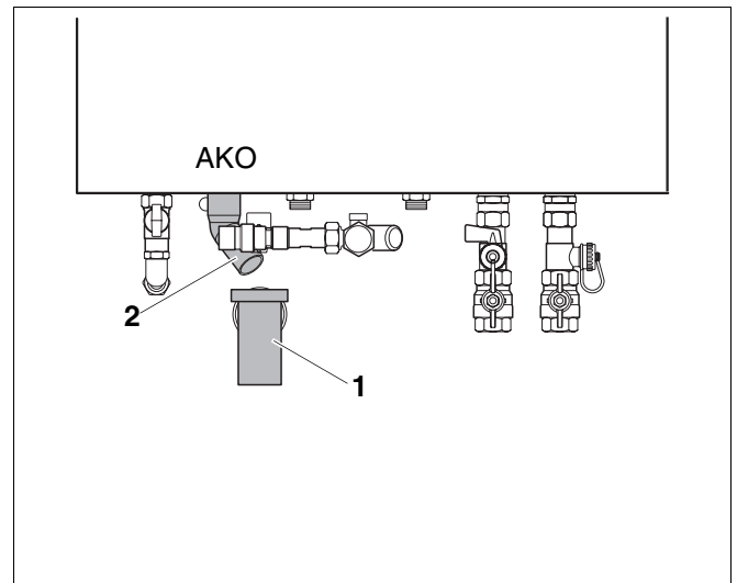
Abb. 19 Trichtersiphon montieren
