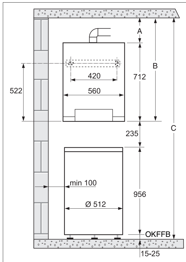
Abb. 15 Äußere Abmessungen bei GB142 mit S120 - OKFFB = Oberkante Fertigfußboden
