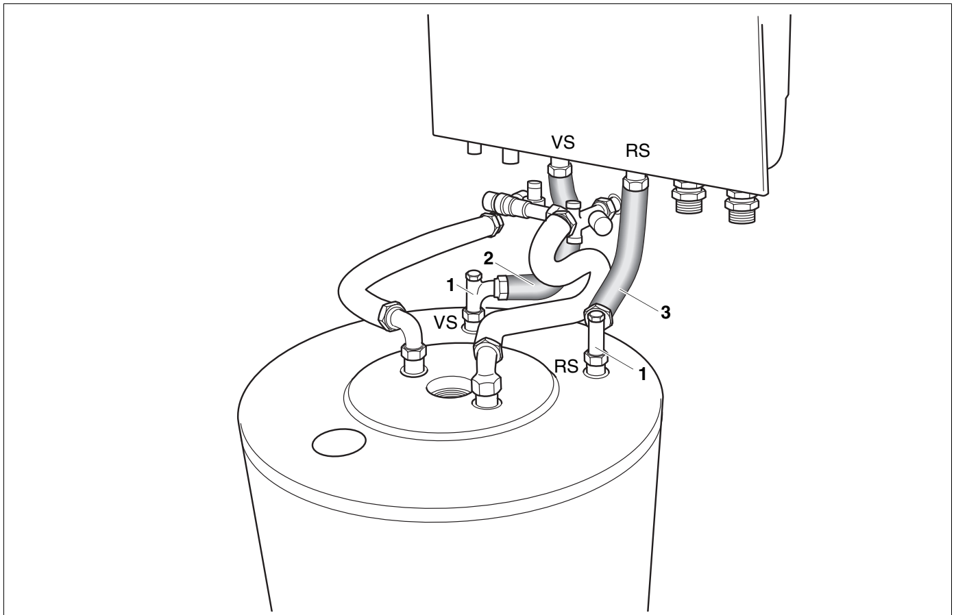
Abb. 16 Montiertes Anschluss-Set U-Flex
