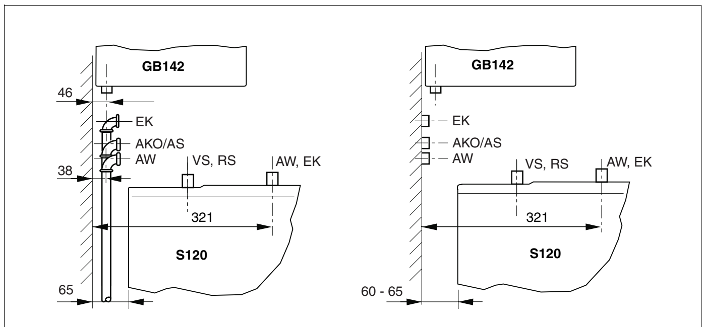
Abb. 14 Abmessungen der Hydraulikanschlüsse, Seitenansicht Aufputzmontage und Unterputzmontage
