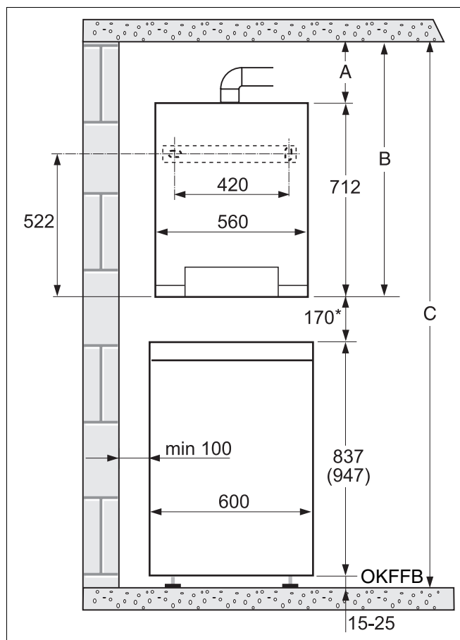
Abb. 5 Abmessungen bei GB142 mit S135 bzw. S160 - Das Maß in der Klammer ist nur für den S160. - OKFFB = Oberkante Fertigfußboden. * Maß 170 ist mit Speicherdeckel
