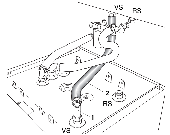
Abb. 8 Well Schlauch an Speichervorlauf montieren
