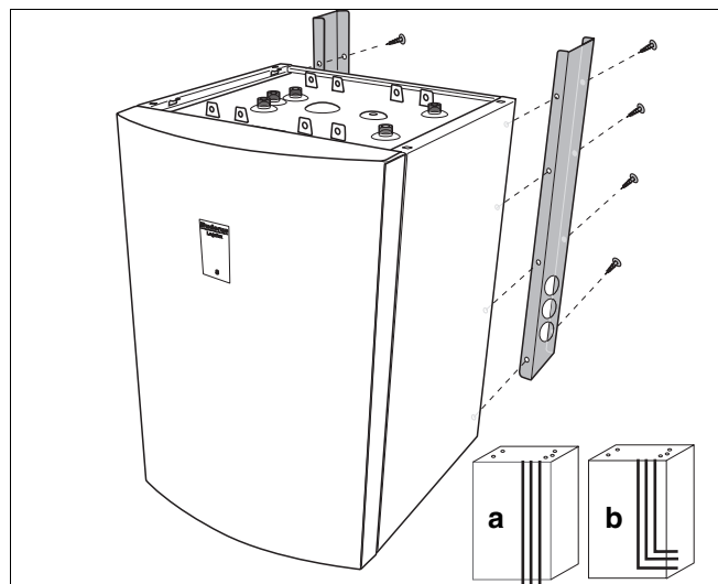
Abb. 10 Seitliche Abdeckung montieren
