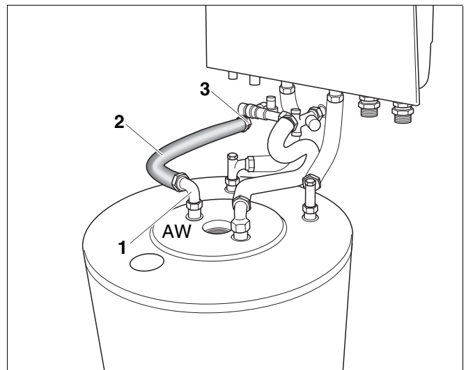
Abb. 28 Warmwasser-Anschlussrohr montieren
