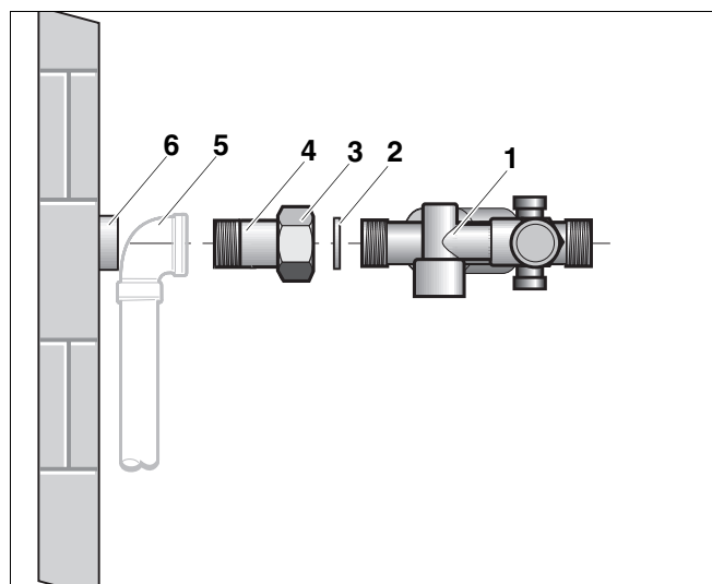
Abb. 11 Sicherheitsgruppe montieren
