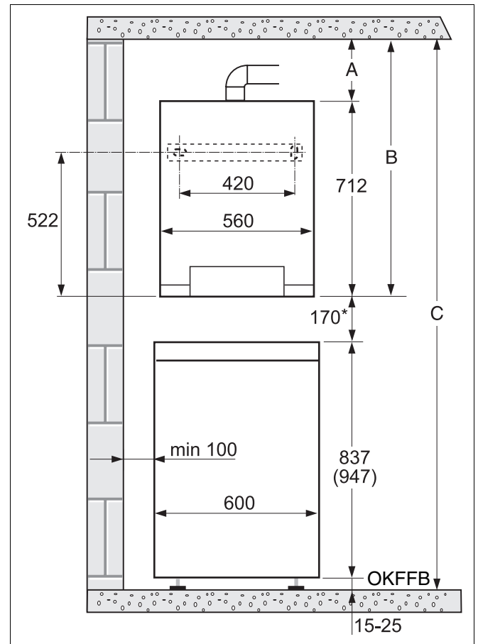
Abb. 8 Abmessungen bei GB142 mit S135 bzw. S160 - Das Maß in der Klammer ist nur für den S160. - OKFFB = Oberkante Fertigfußboden. * Maß 170 ist mit Speicherdeckel
