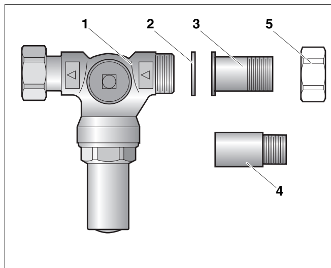
Abb. 2 Lieferumfang Druckminderer U-DM, optional
