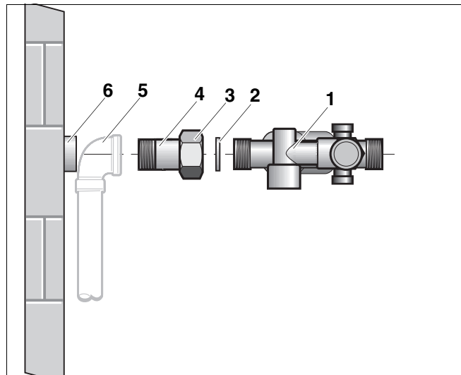
Abb. 23 Sicherheitsgruppe montieren
