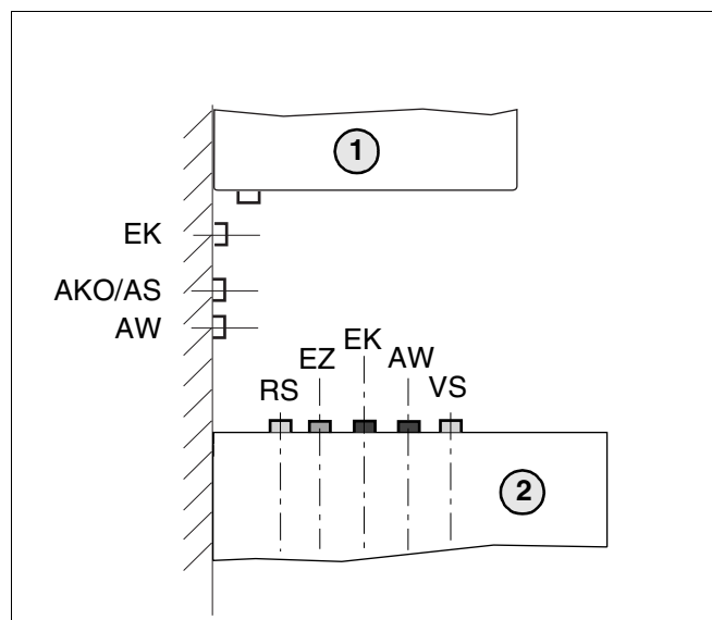
Abb. 6 Abmessungen der Hydraulikanschlüsse S135/S160, Unterputzmontage (Seitenansicht)
