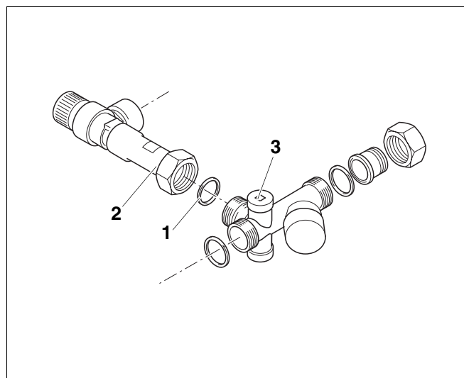
Abb. 24 Sicherheitsgruppe montieren
