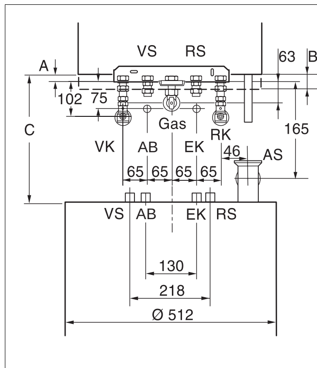
Abb. 7 Abmessung der Hydraulikanschlüsse S120, Vorderansicht
