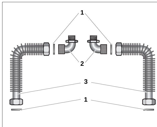
Abb. 1 Lieferumfang heizkreisseitiger Verrohrungssatz U-Flex (Ansicht ohne Wärmeschutz)
