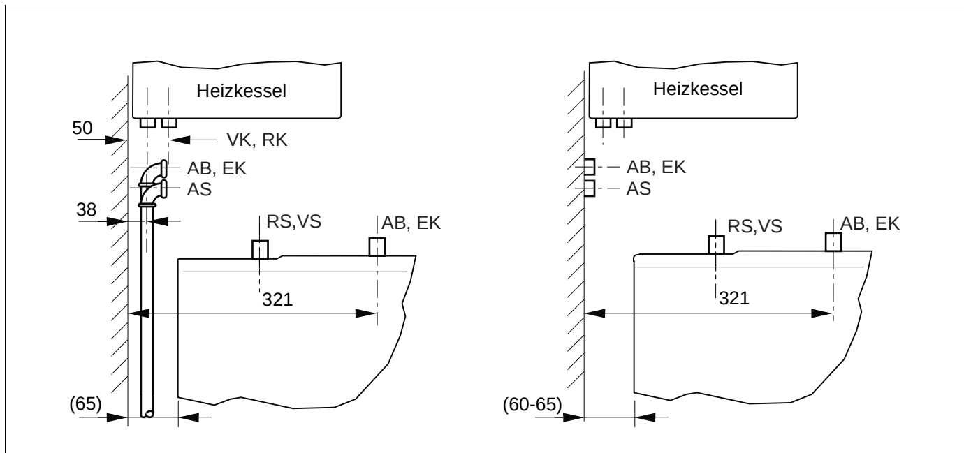
Abb. 6 Abmessungen der Hydraulikanschlüsse, Seitenansicht Aufputzmontage und Unterputzmontage
