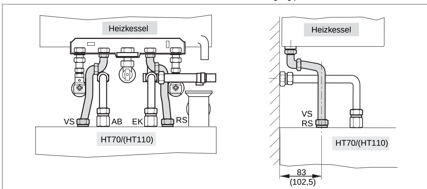
Abb. 9 Verrohrungssatz U-Flex HT70/HT110, Unterputzmontage
