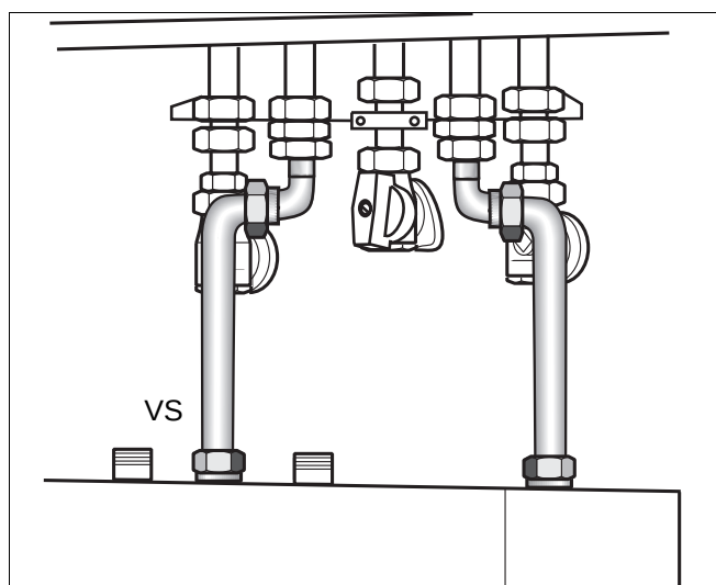
Abb. 13 Well Schlauch Speichervorlauf (Unterputzmontage als Beispiel)
