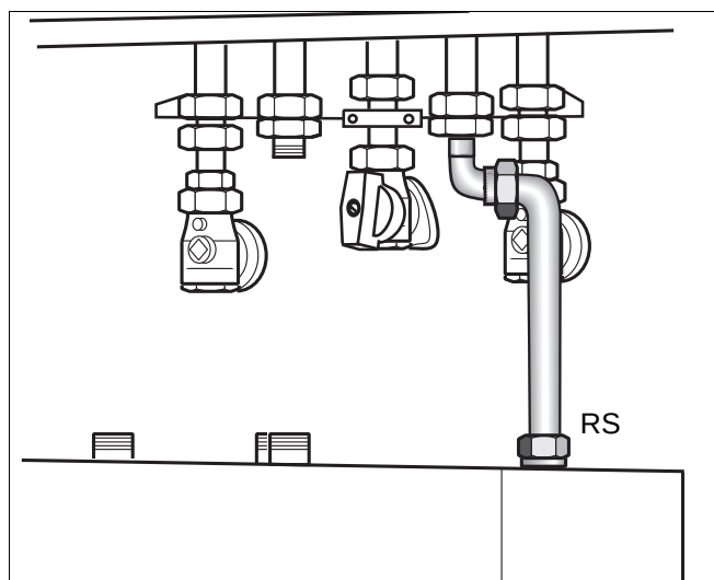
Abb. 12 Well Schlauch Speicherrücklauf (Unterputzmontage als Beispiel)
