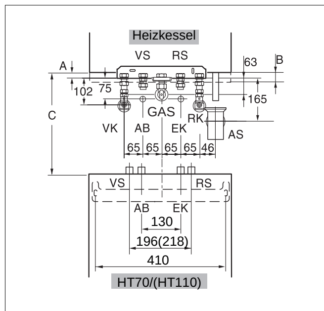
Abb. 3 Abmessungen der Hydraulikanschlüsse, Vorderansicht übereinander
