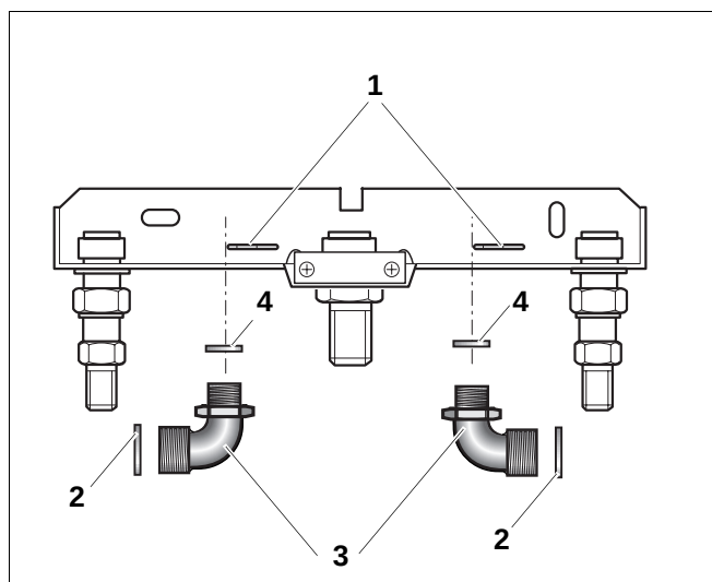
Abb. 11 Abschlusswinkel VS/RS
