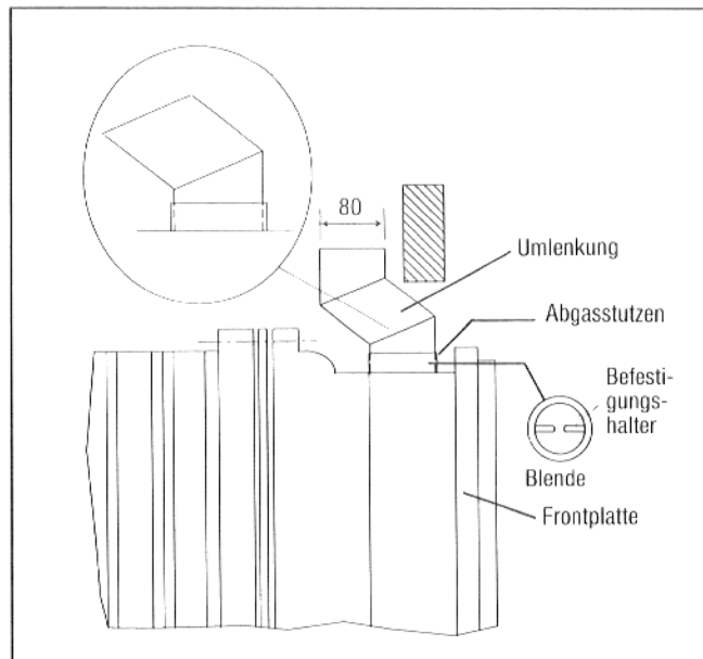
Abb. 2: Vordere Seitenansicht
