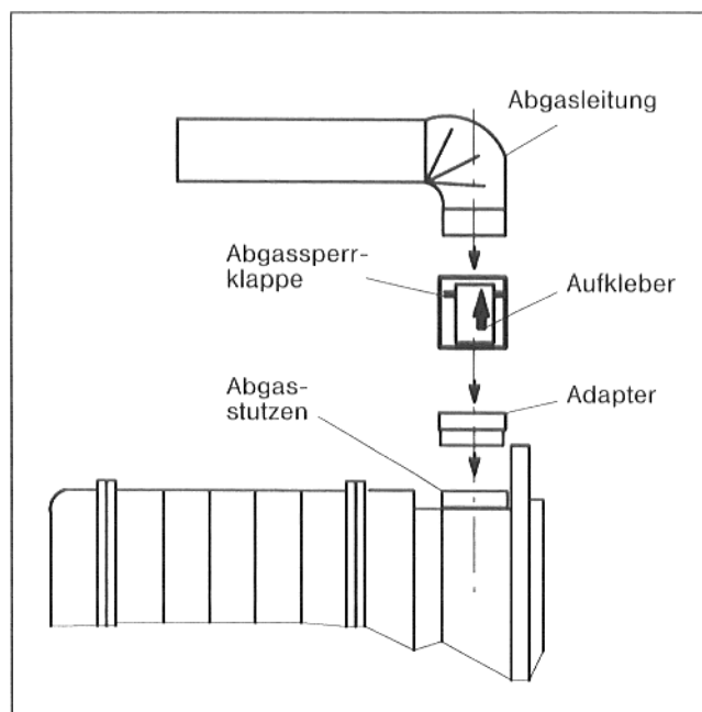
Abb. 15: Einbaulage Abgassperrklappe
