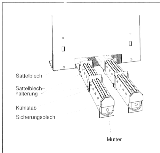
Abb. 8 a: Brennerschild-Rückseite
