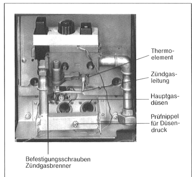
Abb. 7: Heizeinsatznische
