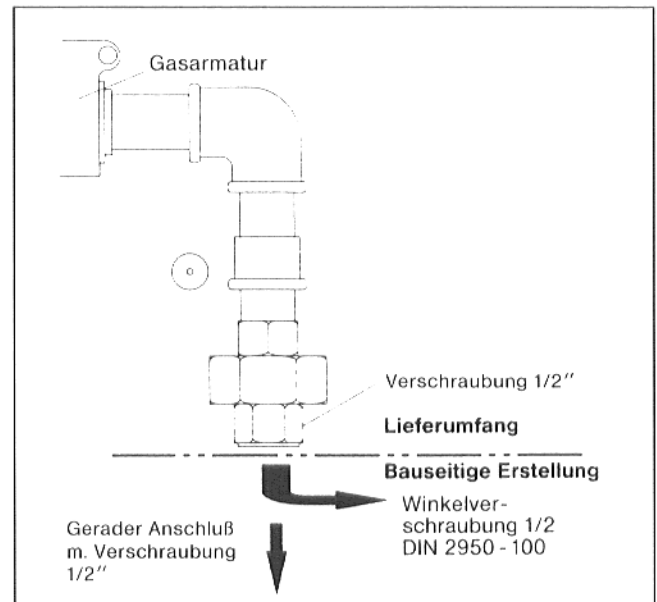
Abb. 1a: Gasanschluß beim H 104 M / H 204 M
