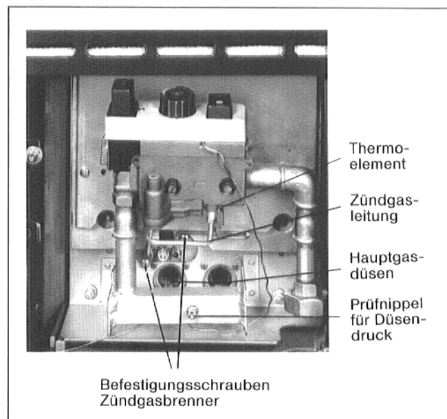
Abb. 7a: Heizeinsatznische
