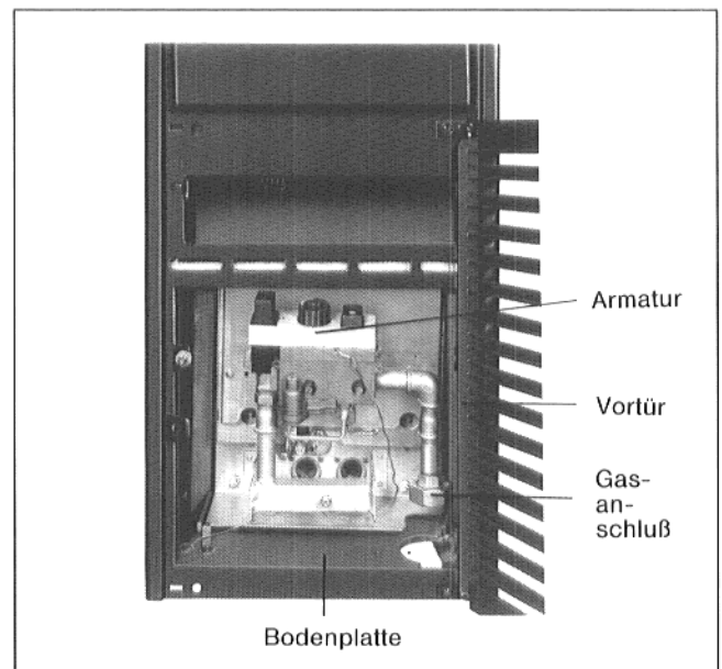
Abb. 1: Heizeinsatz mit geöffneter Vortür
