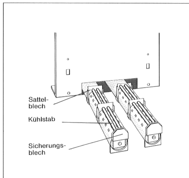
Abb. 10: Brennerschild; Rückseite mit Brennstäben
